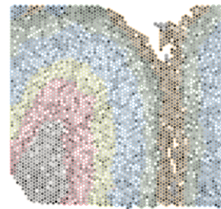
FAIM2
