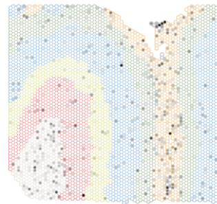
GAD1
