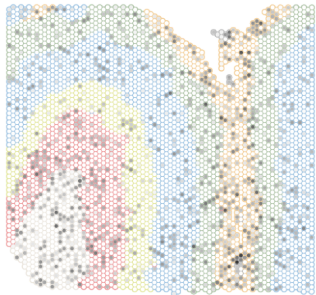
PRKAR1A
