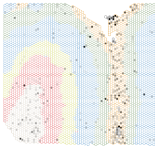
APOE
