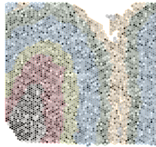
APLP1
