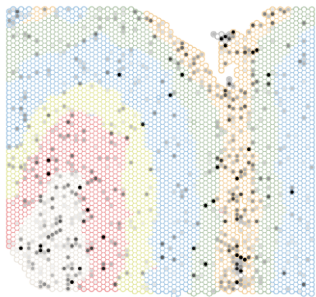
MT1X
