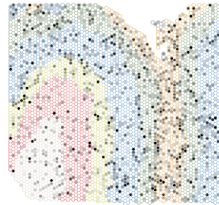
FTL
