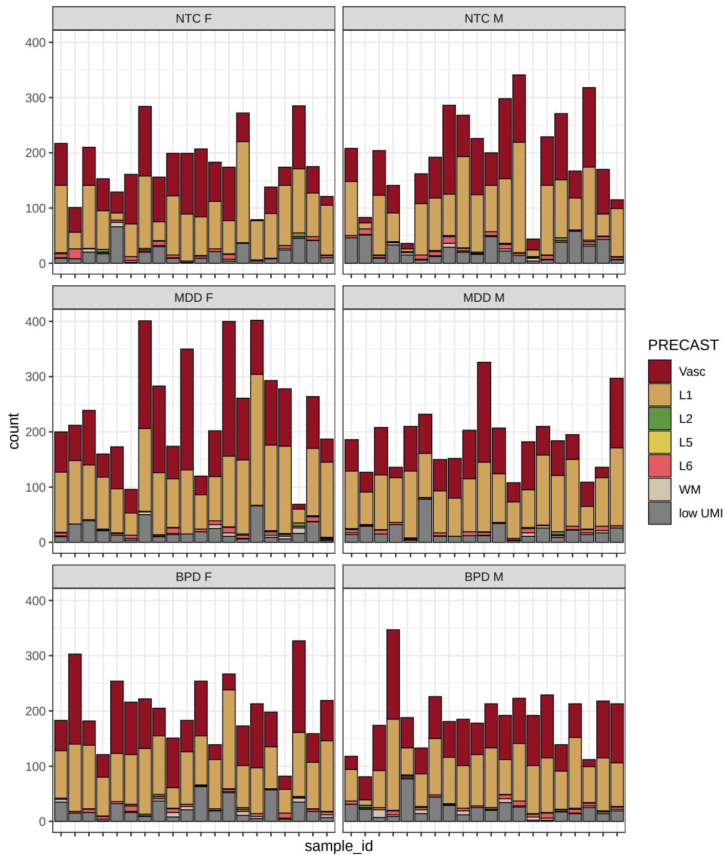
Only Seurat pc20 Micro.Vasc
