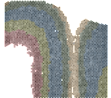
BPD F
