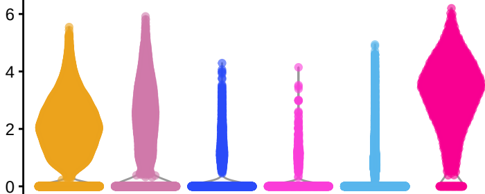
DRD1
