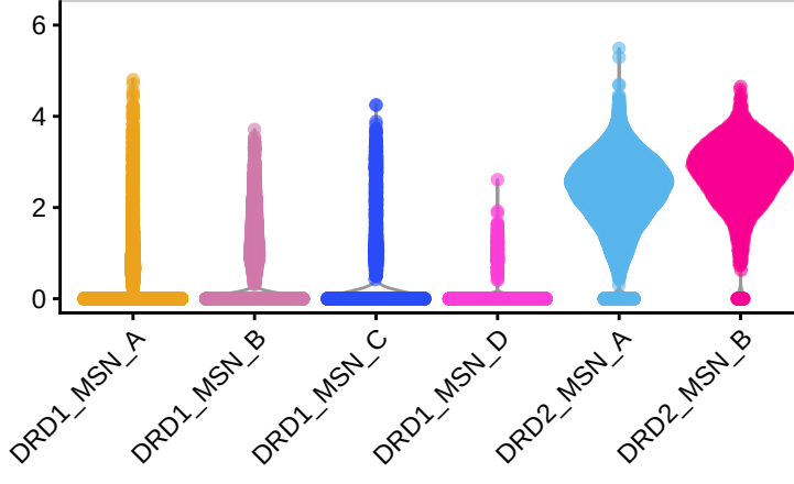
DRD2
