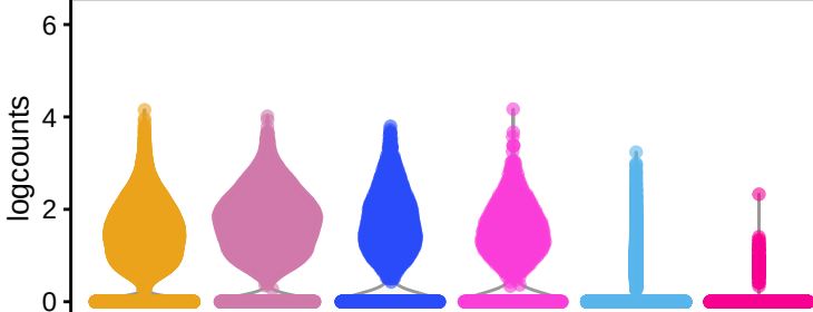
DRD2
