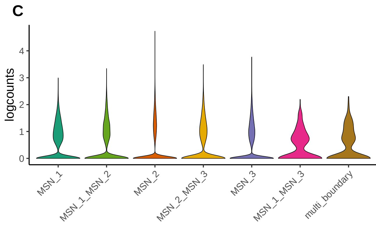
CALB1
