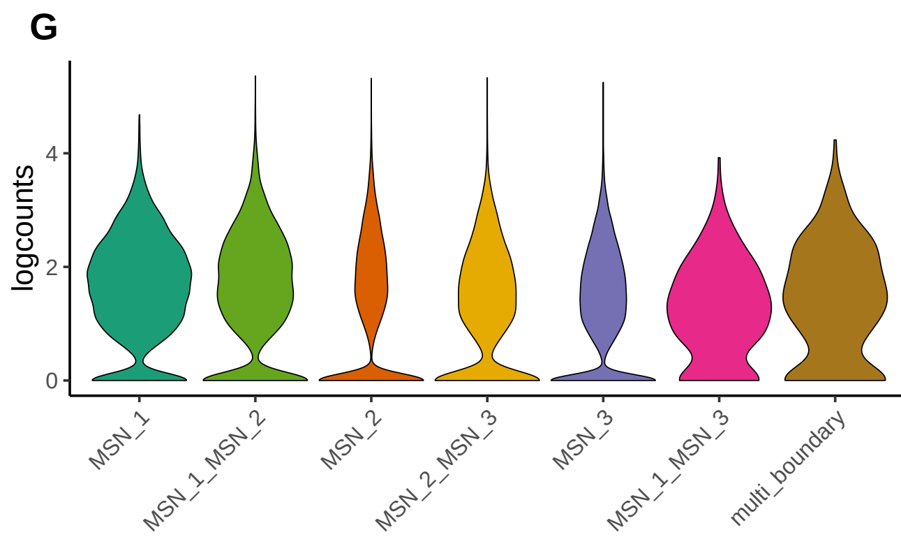
ADORA2A
