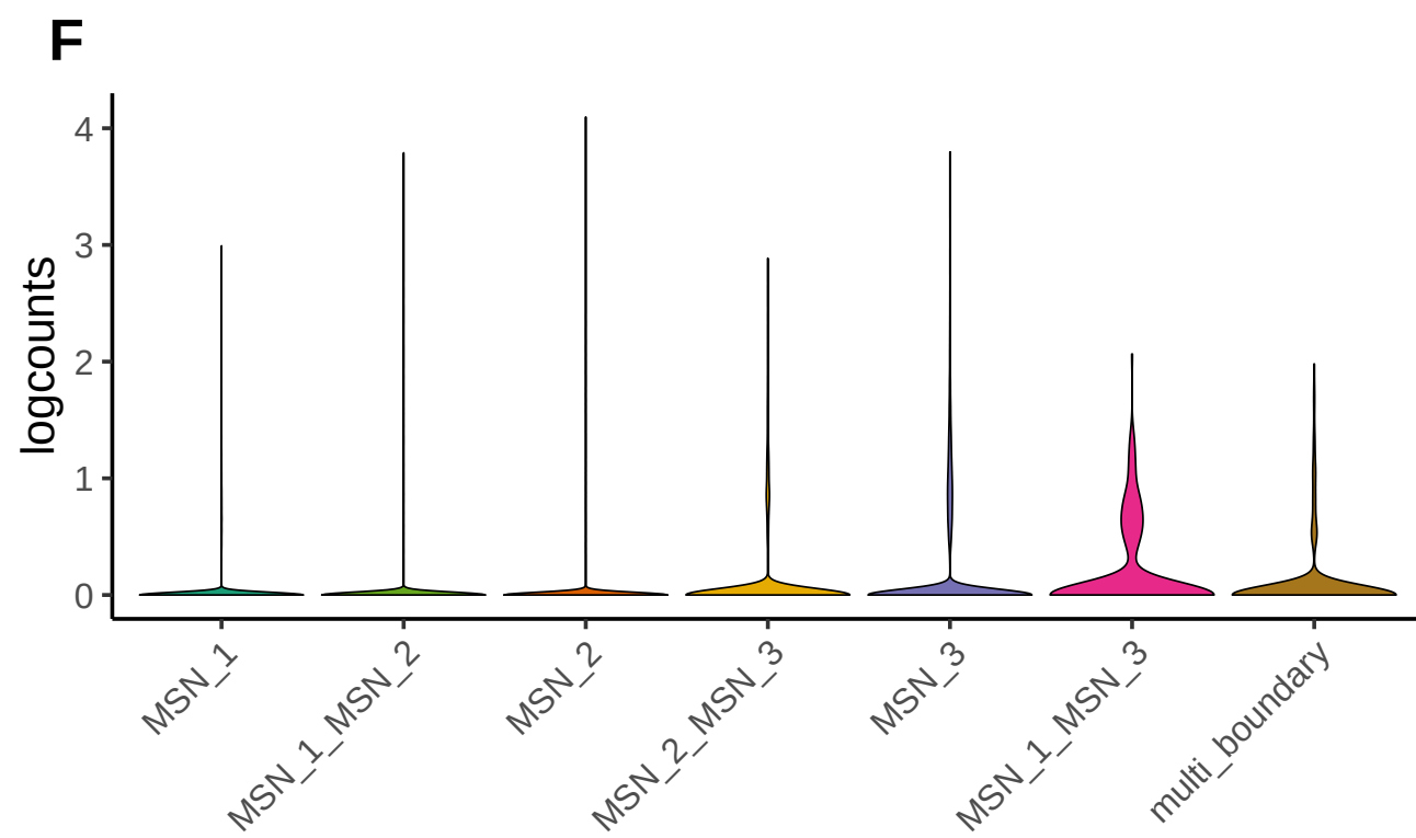
PDYN
