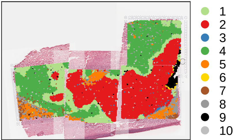
Random start: 4
