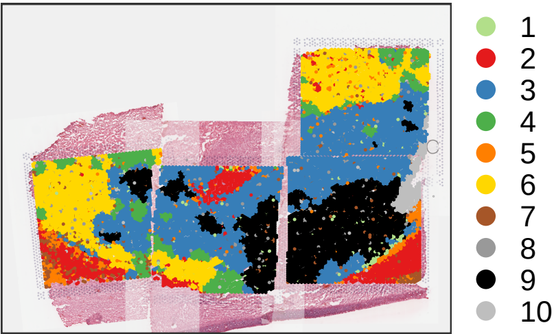
Random start: 5
