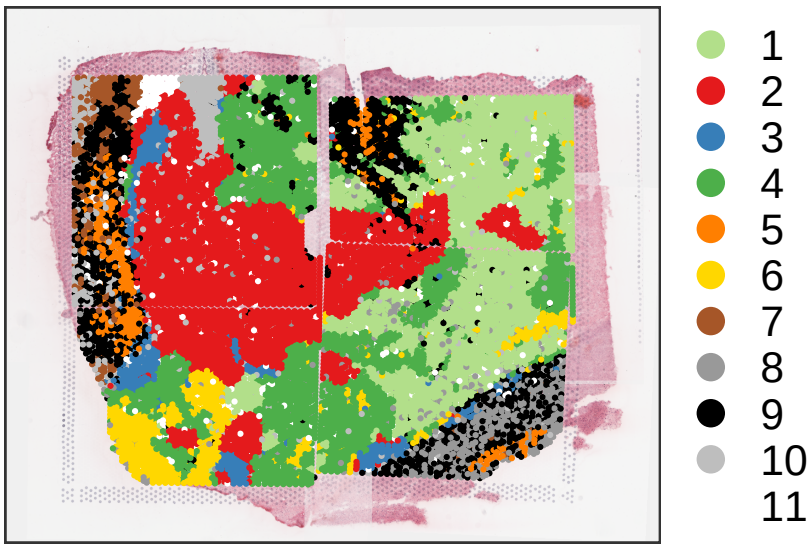
Random start: 4
