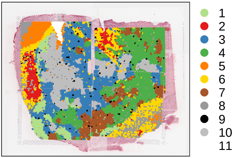
Random start: 5
