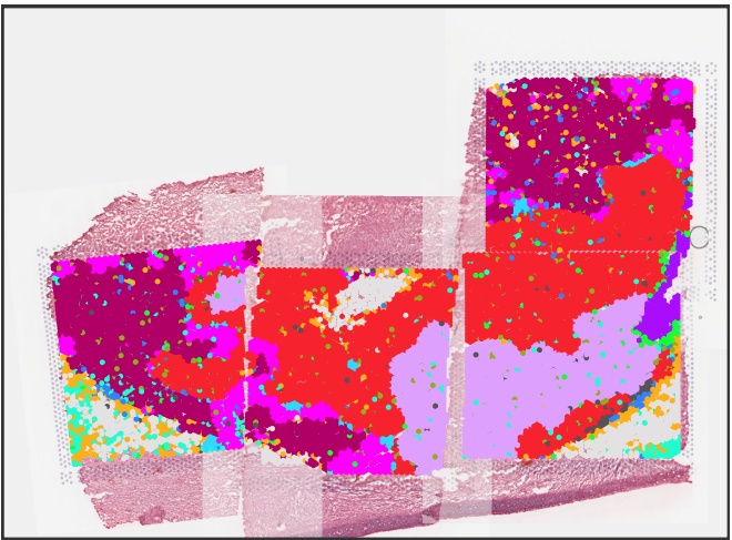
Random start: 5
