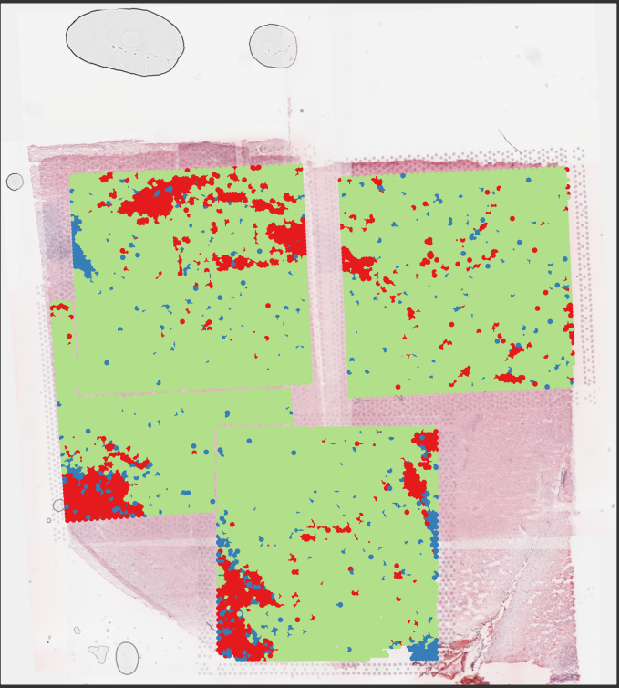
Random start: 5
