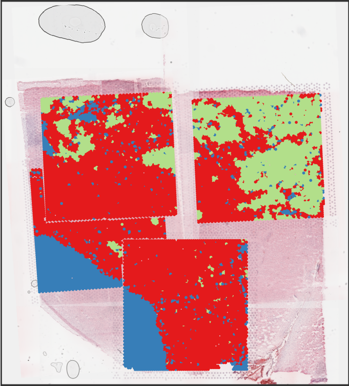
Random start: 4
