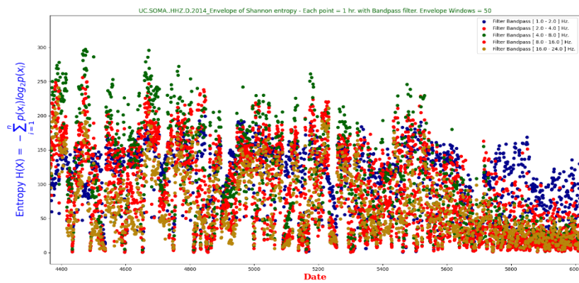
Fig. 79 Acercamiento (ZOOM intervalo de 4400-6000 en el recuadro azul punteado, figura 78), Gráfica (puntos) de la comparación de las envolturas tomando los 5 grupos de valores del filtro paso-banda (Bandpass).
