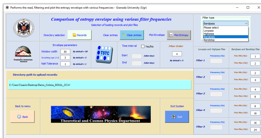
Fig. 75 Interfaz del módulo de las entradas del módulo de cálculo y comparación de envolventes de la Entropía de Shannon, utilizando varias frecuencias de filtros.
