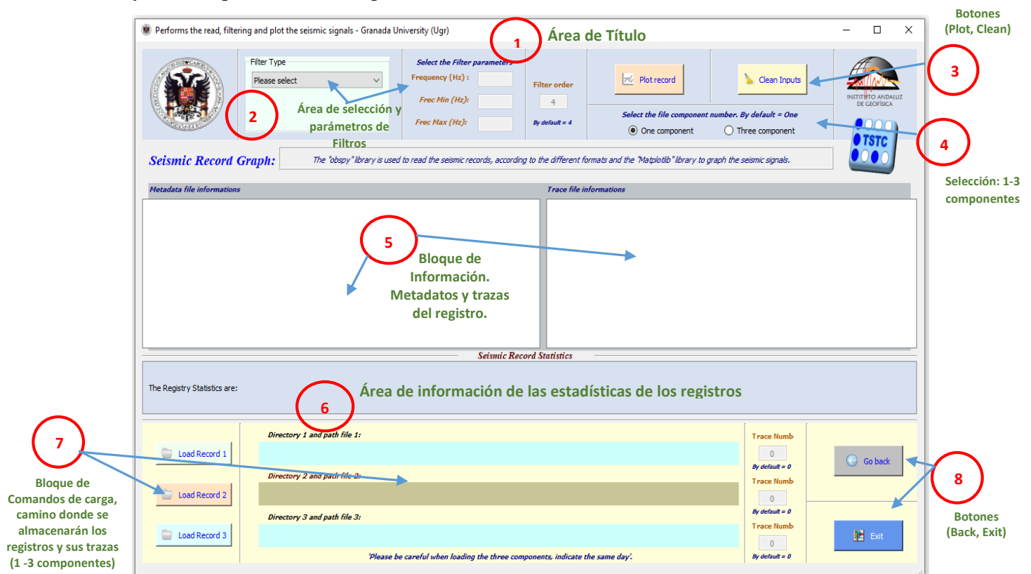
Fig. 7 Interfaz del módulo de lectura, filtrado y gráfica de registros y elementos que la componen.
