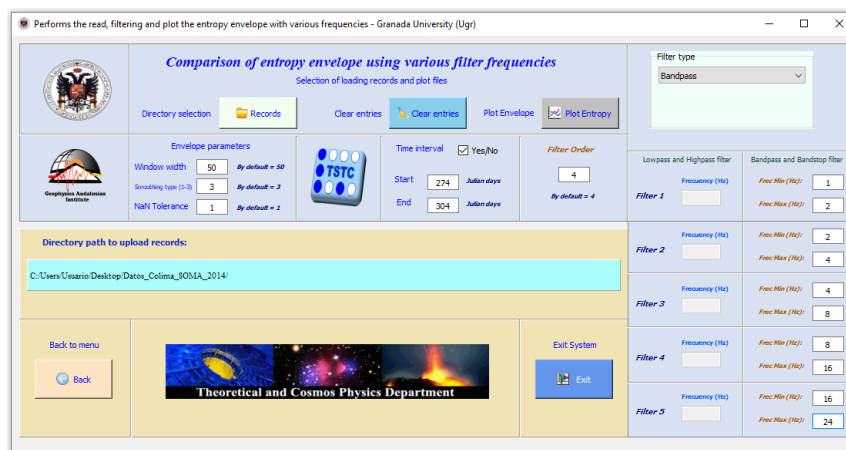
Fig. 80 Interfaz del módulo del módulo de cálculo y comparación de envolturas, con los parámetros por defecto (50,3,1) de la Entropía de Shannon, utilizando varias frecuencias de filtros y un intervalo de tiempo de 274 a 304 días julianos, lo que corresponde al mes de Octubre (Año no bisiesto).
