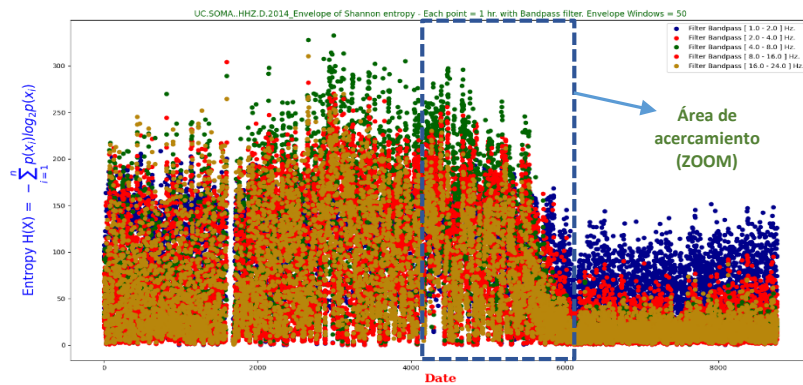
Fig. 78 Gráfica (puntos) de la comparación de las envolturas tomando los 5 grupos de valores del filtro paso-banda (Bandpass).
