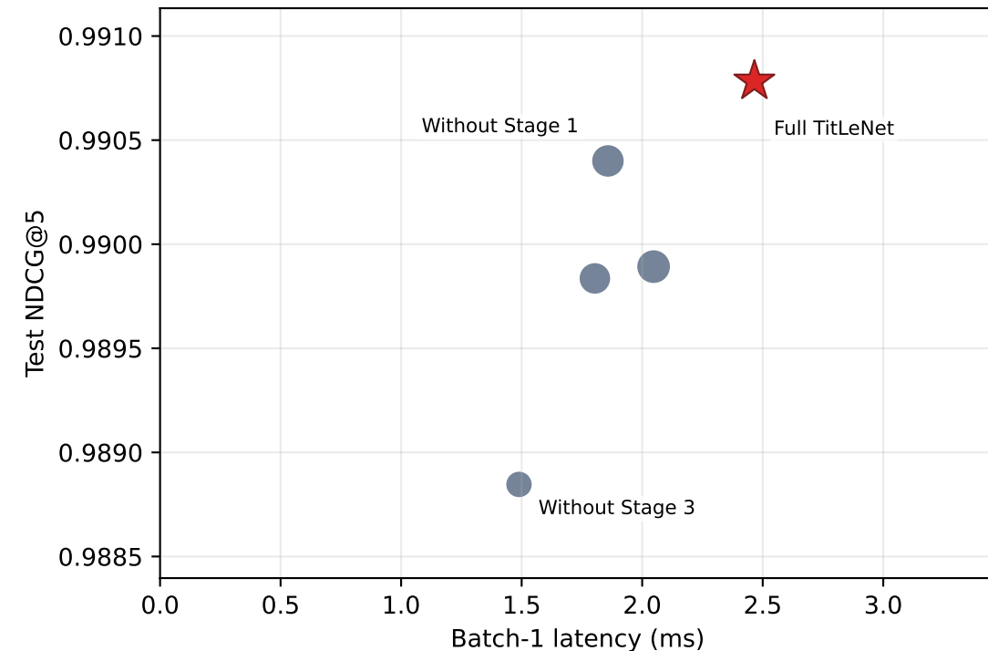
(d) Latency vs Test NDCG@5
