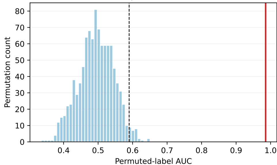
donor_expression_pca p=0.0010
