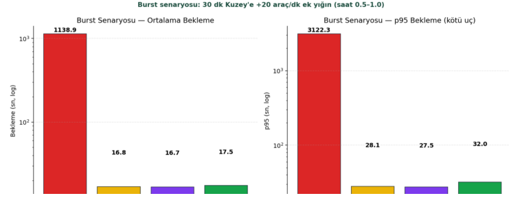
Şekil B.5: Ani Talep Senaryosu sekmesi. Sabit zamanlı yöntemin uyarlanı yönteme göre 67 kat daha kötü performans gösterdiği logaritmik ölçekli karşılaştırma grafiği.
