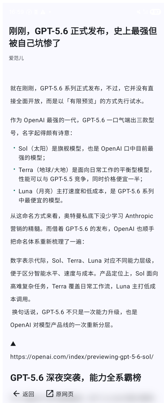
图 4: 文章阅读页
