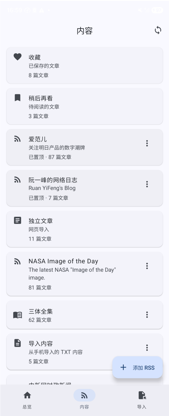
图 2: 内容管理页
