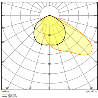
FL PFM 200W 4000K ASYM 55x110 BK
