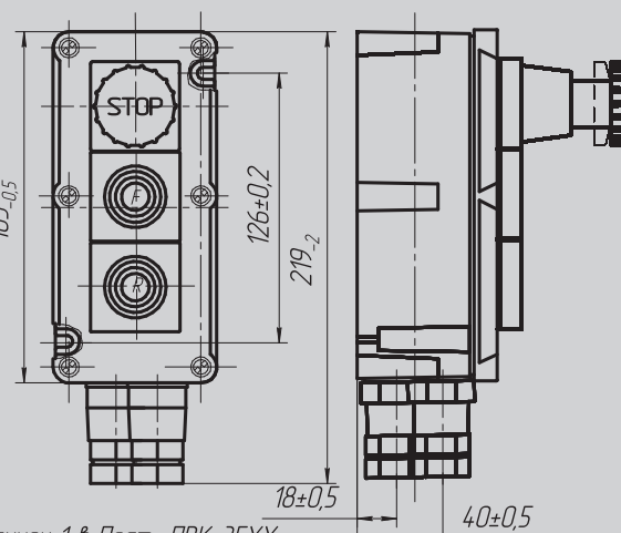
Рисунок 1 б Пост ПВК-35ХХ Остальное см. рис. 1 а и 1 б.
