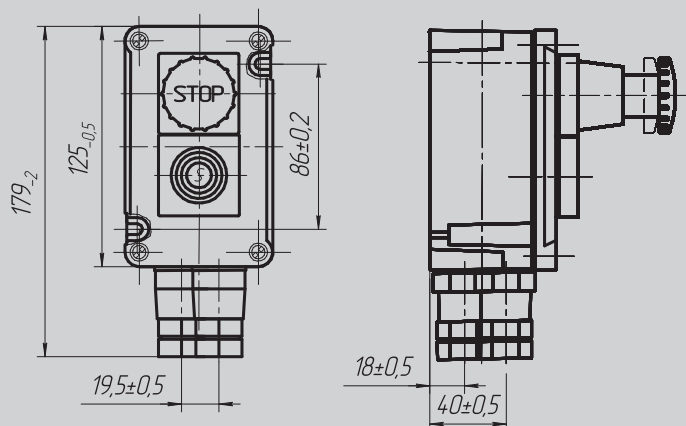
Рисунок 1 в Пост ПВК - 25ХХ Остальное - см. рис. 1 а
