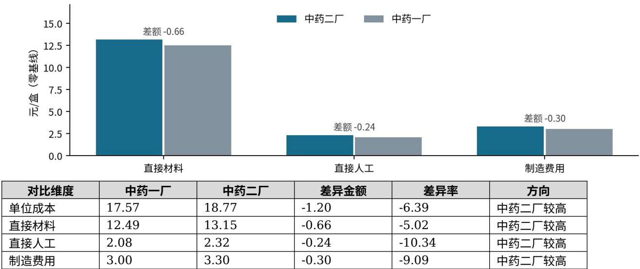
图 | 六味地黄胶囊 · 2026-06 | 跨厂三要素（中药一厂-中药二厂，以中药二厂为分母）
