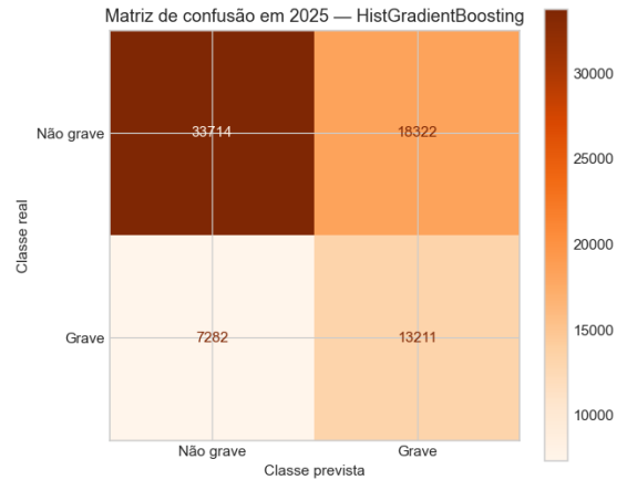
Figura 3: Matriz de confusão do modelo escolhido.
