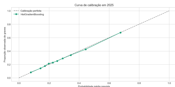
Figura 6: Curva de calibração no teste.
