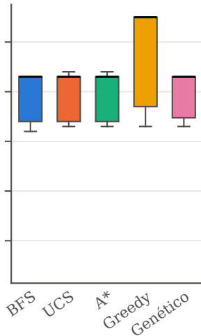
Mapa 2: laberinto
