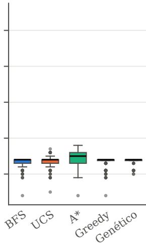
Mapa 3: abierto
