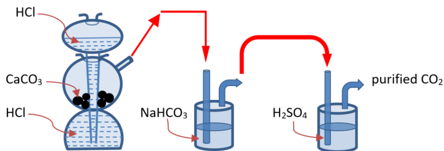
Kipps apparatus
