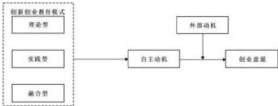
图 3-1 理论模型图
