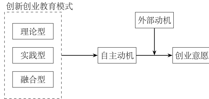
图 3-1 理论模型图
