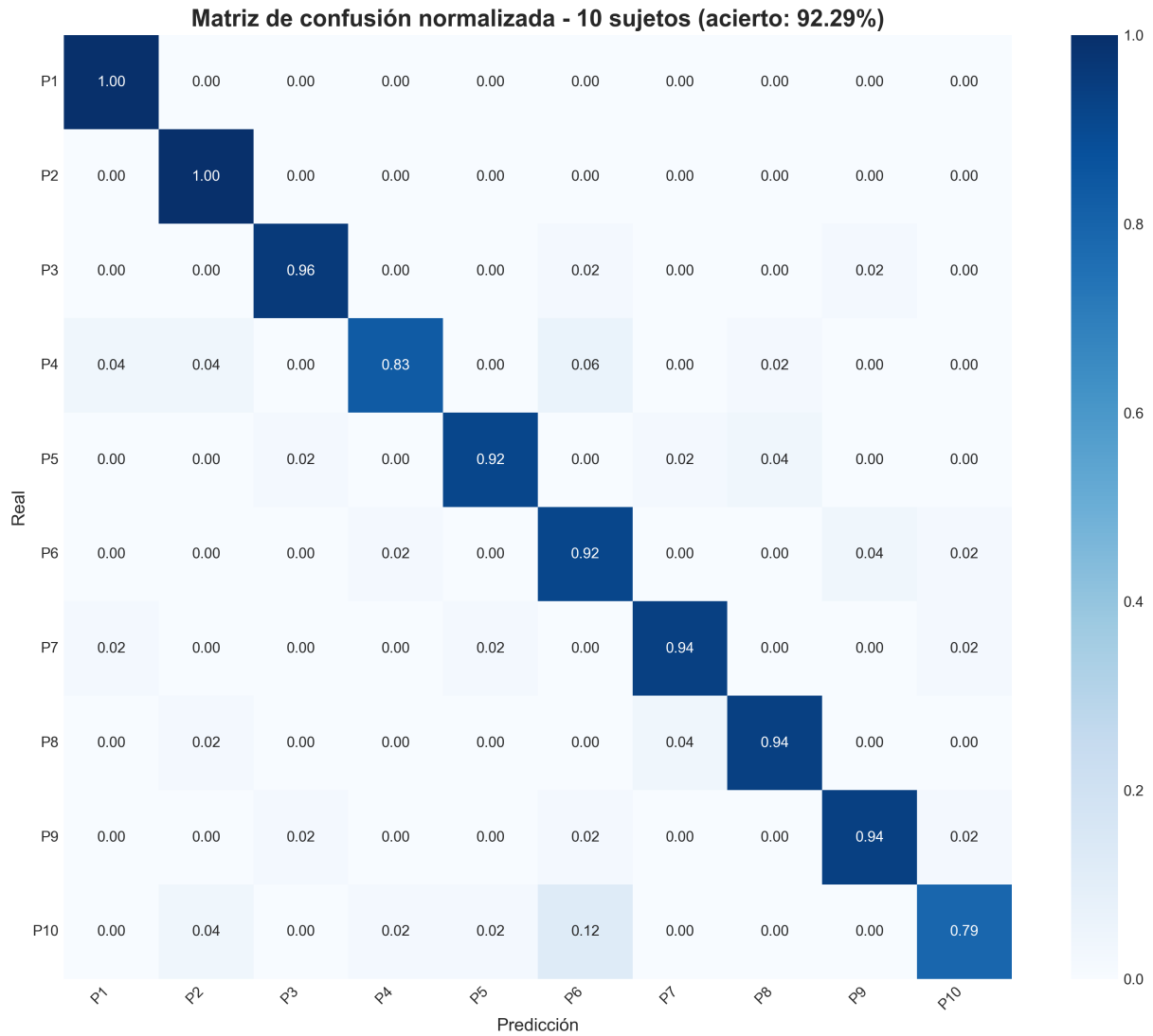
Figura 4.19: Matriz de confusión normalizada — Random Forest con k = 10 sujetos (exactitud: 92.29 %, confianza media en aciertos: 0.669). La exactitud se mantiene estable respecto a k = 5 a pesar de duplicar el número de clases, evidenciando la robustez del sistema en el régimen de escalabilidad moderada.
