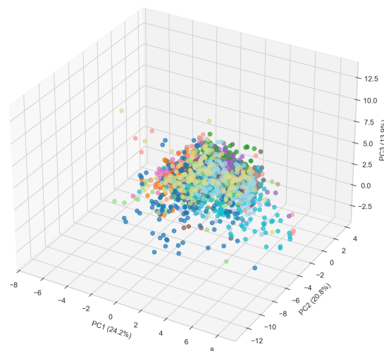
Figura 4.13: Proyección tridimensional de los datos sobre las tres primeras componentes principales (PC1, PC2 y PC3). Aunque se incorpora una dimensión adicional, el solapamiento entre sujetos persiste, confirmando que la varianza explicada por estas componentes es insuficiente para una discriminación fiable.
