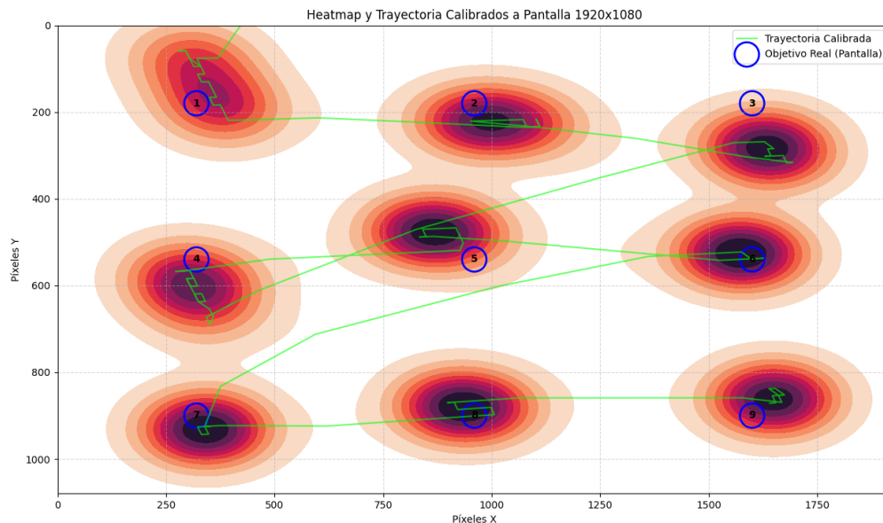
Figura 4.22: Mapa de calor de la mirada corregida mediante la matriz de homografía para la cuadrícula 3 \times 3 . Las zonas rojas (alta densidad) coinciden con la ubicación de los 9 puntos de calibración, demostrando que el usuario mantuvo fijaciones estables sobre los objetivos. Las líneas tenues entre clústeres representan las trayectorias sacádicas de transición.
