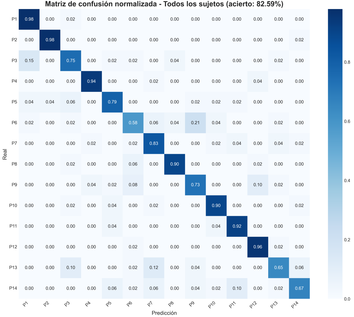
Figura 4.20: Matriz de confusión normalizada — Random Forest con k = 14 sujetos (exactitud: 82.59 %, \bar{F1} = 0.823 \pm 0.087 ). La diagonal dominante confirma el alto rendimiento global del sistema. Las confusiones fuera de la diagonal se concentran en P6 y P9, sujetos cuyo perfil biométrico presenta mayor solapamiento inter-clase.
