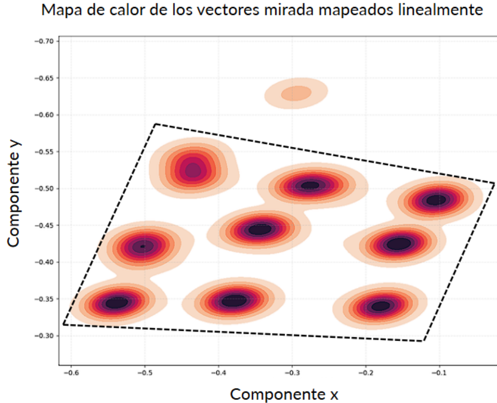
Figura 4.21: Distribución espacial de las coordenadas oculares proyectadas mediante un mapeo estrictamente lineal. La ausencia de corrección homográfica evidencia el error de paralaje y la deformación geométrica entre el plano de la cámara y el plano de la pantalla.
