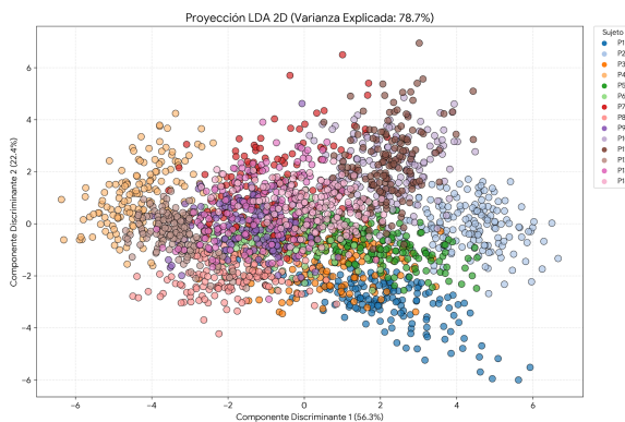
Figura 4.8: Proyección en 2D (LD1 vs LD2)
