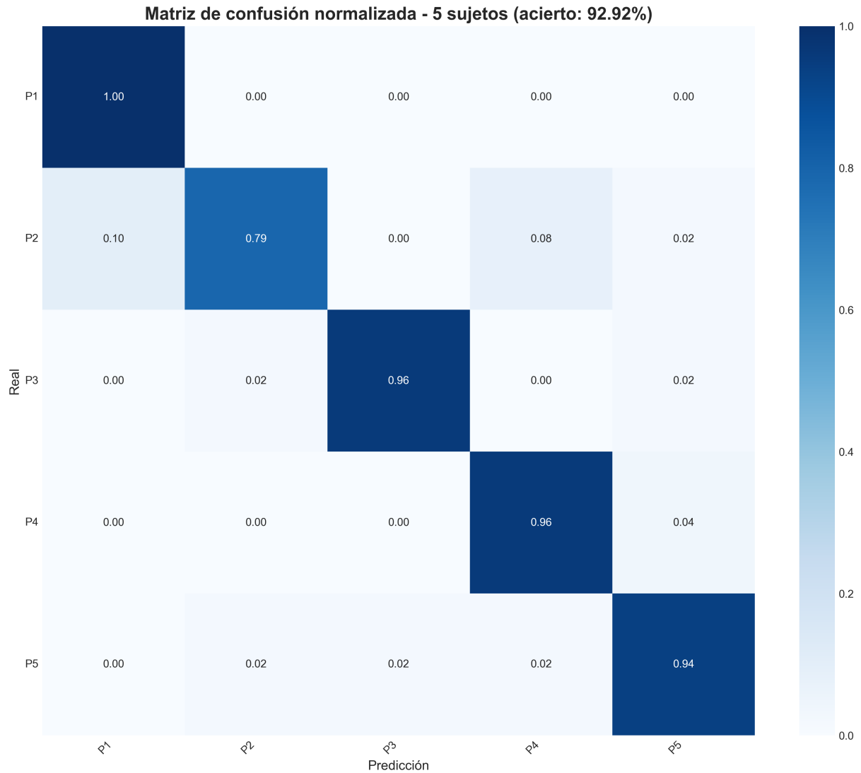
Figura 4.18: Matriz de confusión normalizada — Random Forest con k = 5 sujetos (exactitud: 92.92 %, confianza media en aciertos: 0.821). La diagonal prácticamente unitaria refleja la alta separabilidad del espacio de características cuando el número de clases es reducido.
