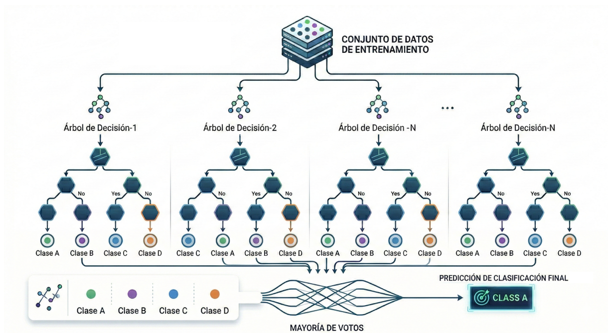
Figura 2.3: Arquitectura del clasificador Random Forest . El diagrama ilustra el mecanismo de ensamblaje: múltiples árboles de decisión ( Tree_1 \dots Tree_n ) procesan la entrada independientemente. La clase final se determina mediante la mayoría de votos ( Majority Voting ), lo que reduce la varianza y mejora la generalización del modelo.
