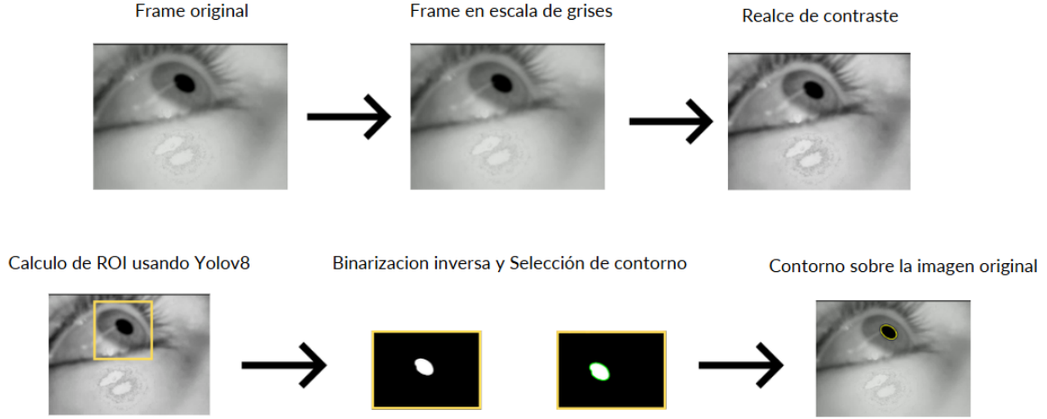
Figura 3.8: Pipeline de procesamiento de imagen implementado. La secuencia muestra: (Arriba) Mejora de la imagen mediante escala de grises y realce de contraste CLAHE. (Abajo) Detección de la ROI con YOLOv8, binarización inversa adaptativa y superposición final del contorno elíptico ajustado sobre la imagen original.
