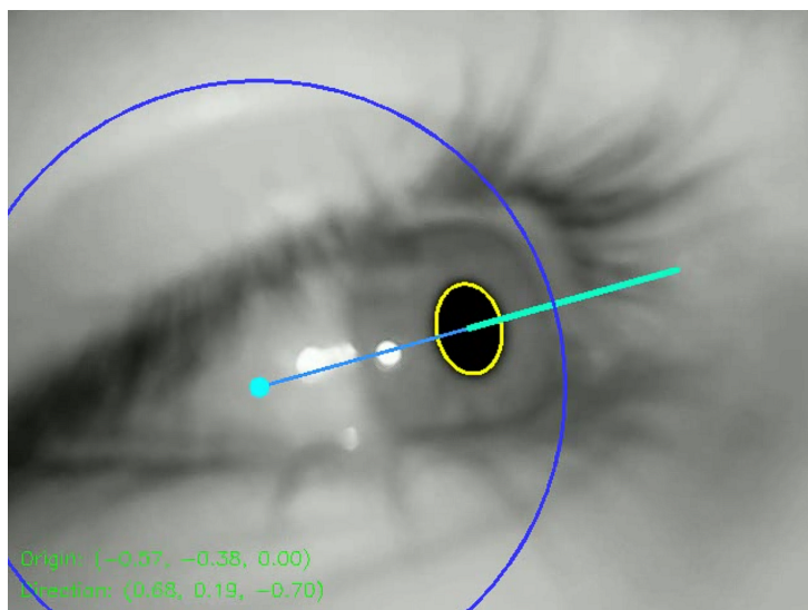
Figura 2.2: Método de pupila oscura y vector de dirección de la mirada. La pupila aparece como una región oscura debido a la absorción de luz infrarroja por la retina.
