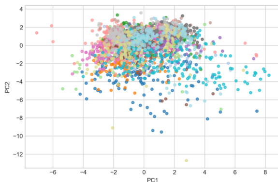
Figura 4.12: Proyección de los datos en las dos primeras componentes principales (PC1 y PC2), que en conjunto explican aproximadamente el 20 % de la varianza total. Se observa un fuerte solapamiento entre las clases, lo que evidencia la limitada separabilidad lineal del espacio biométrico original.
