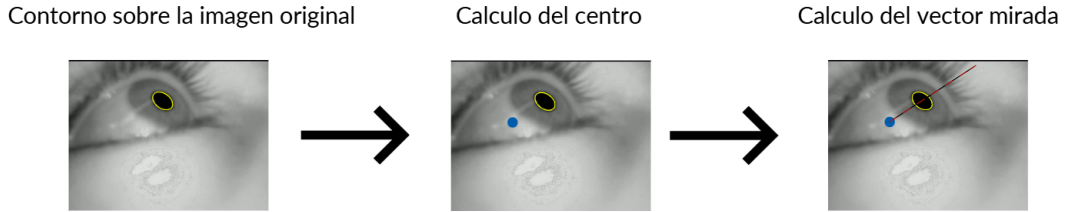
Figura 3.12: Esquema del pipeline de estimación del vector de mirada. (Izquierda) Segmentación del contorno pupilar y ajuste de elipse. (Centro) Centro del Modelo c (punto azul) estimado por convergencia de ejes normales respecto al centroide de la pupila (punto rojo). (Derecha) Vector de mirada \hat{g} (línea roja) resultante de la proyección esférica, cuya orientación en el espacio 3D determina la dirección de fijación del sujeto.
