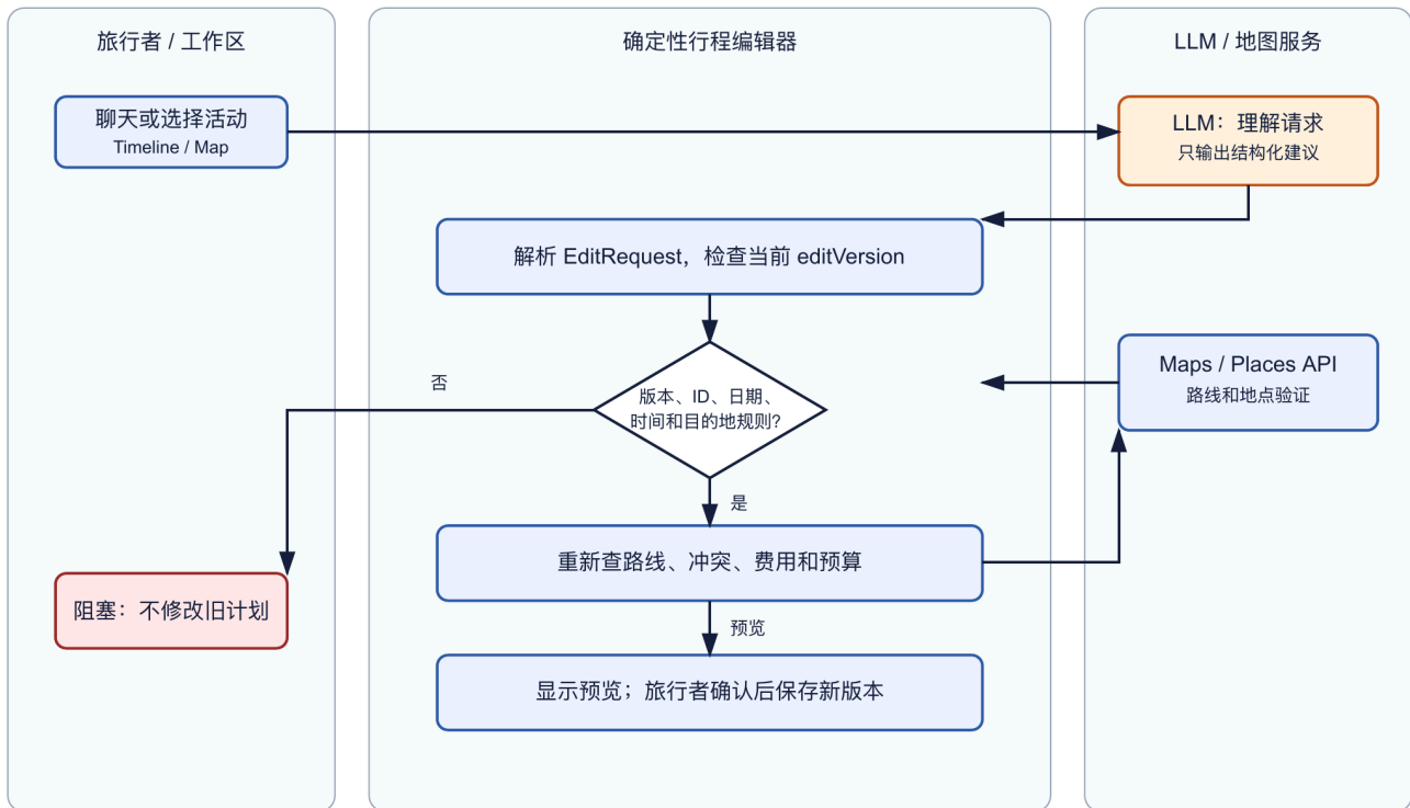
UC-E1 活动图：编辑行程
