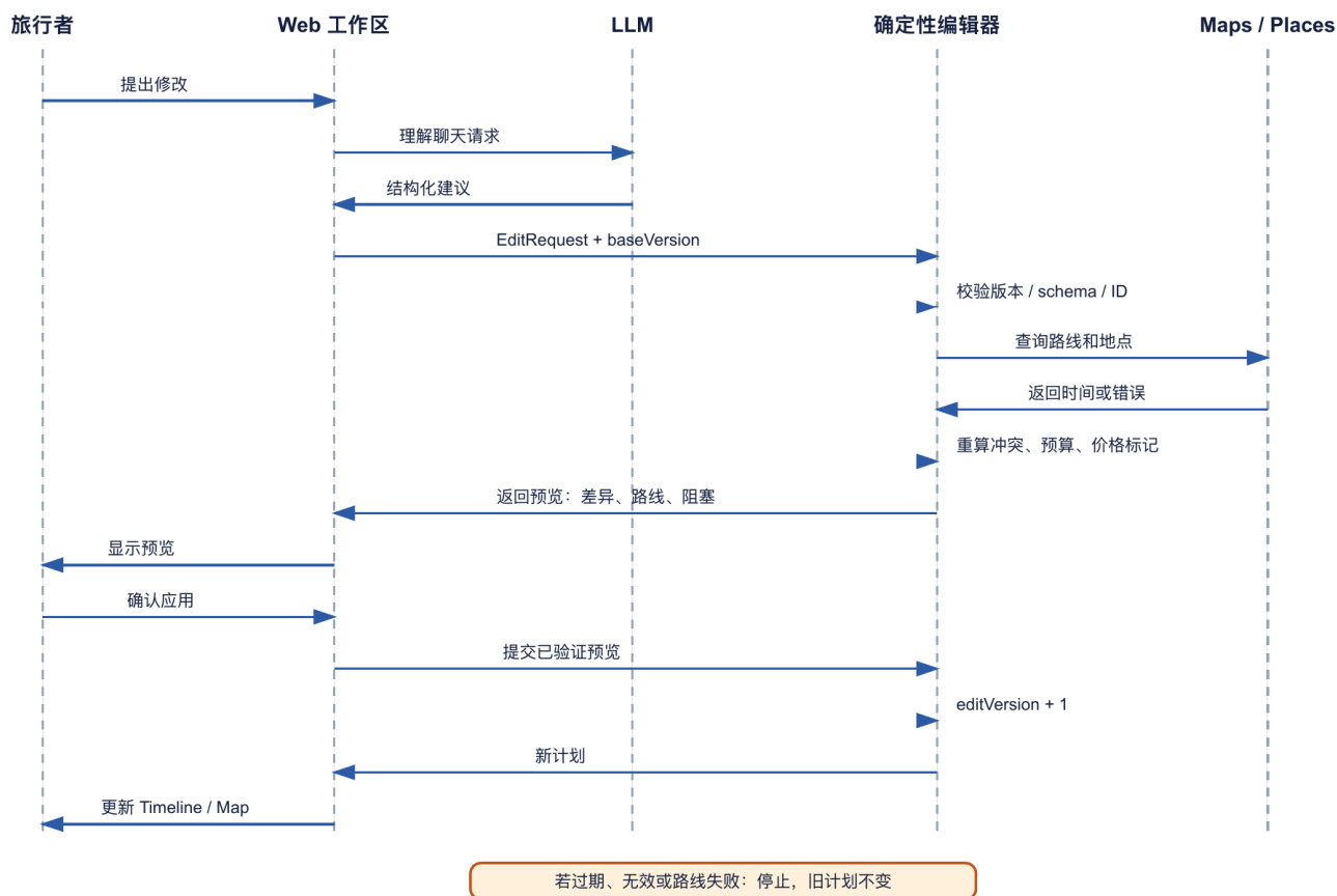
UC-E1 时序图：预览并应用行程编辑
