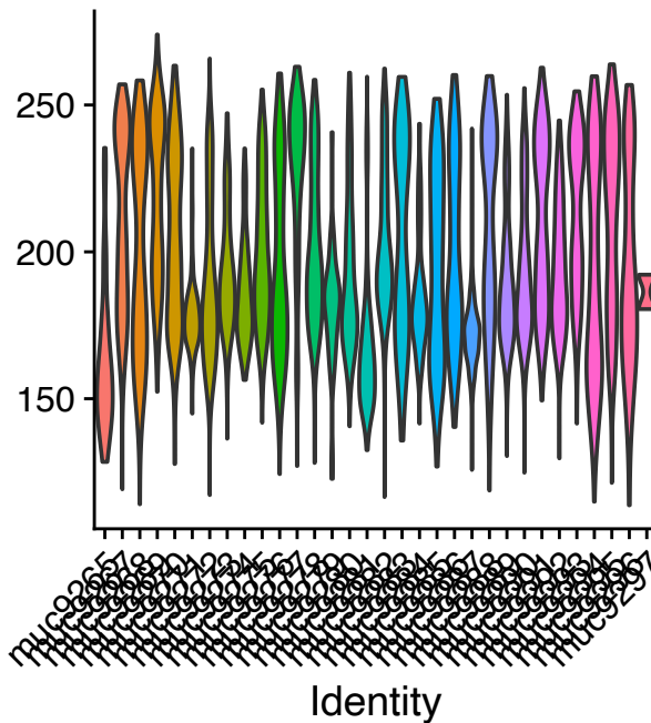
n_counts
