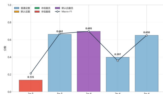
图 7 学习率消融
