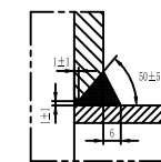
板板示意图
