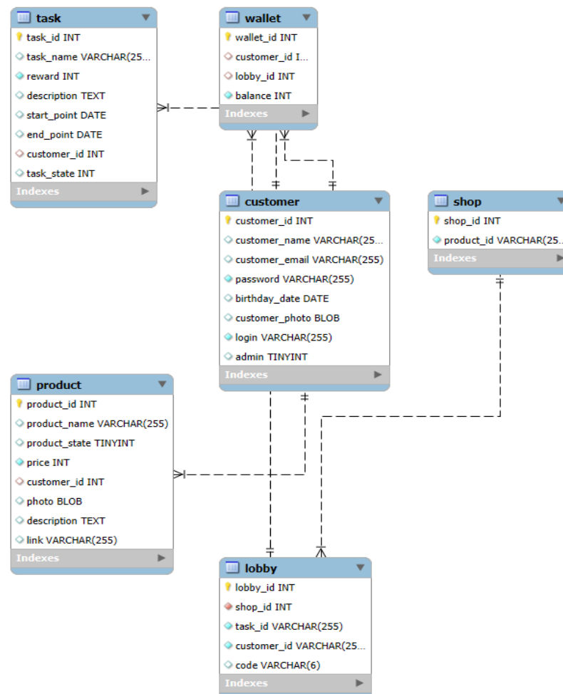
Рисунок 6 — ER-диаграмма.
