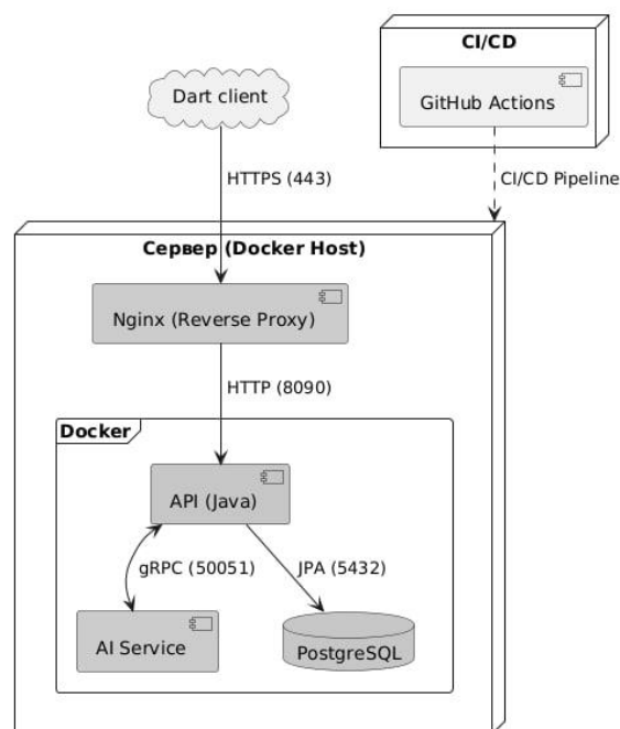
Рисунок 1 — Схема развертывания.
