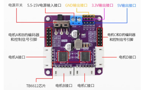
四路电机控制引出
