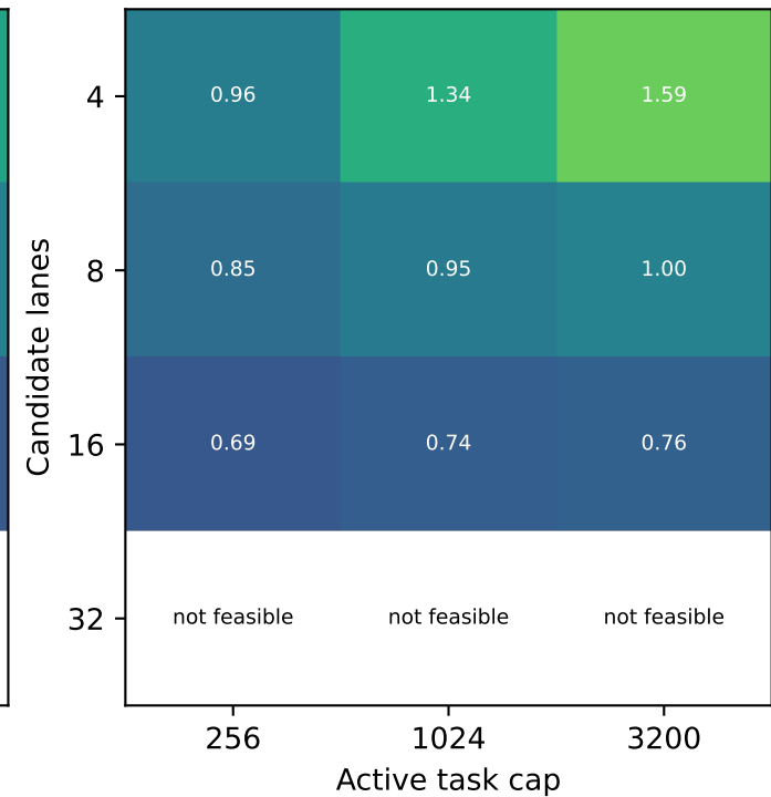
TSP100 / cohort g50
