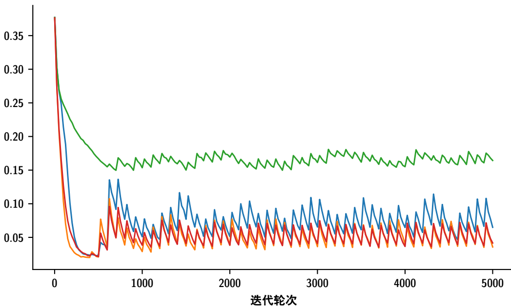
2-opt 后路径之间的边不一致率
