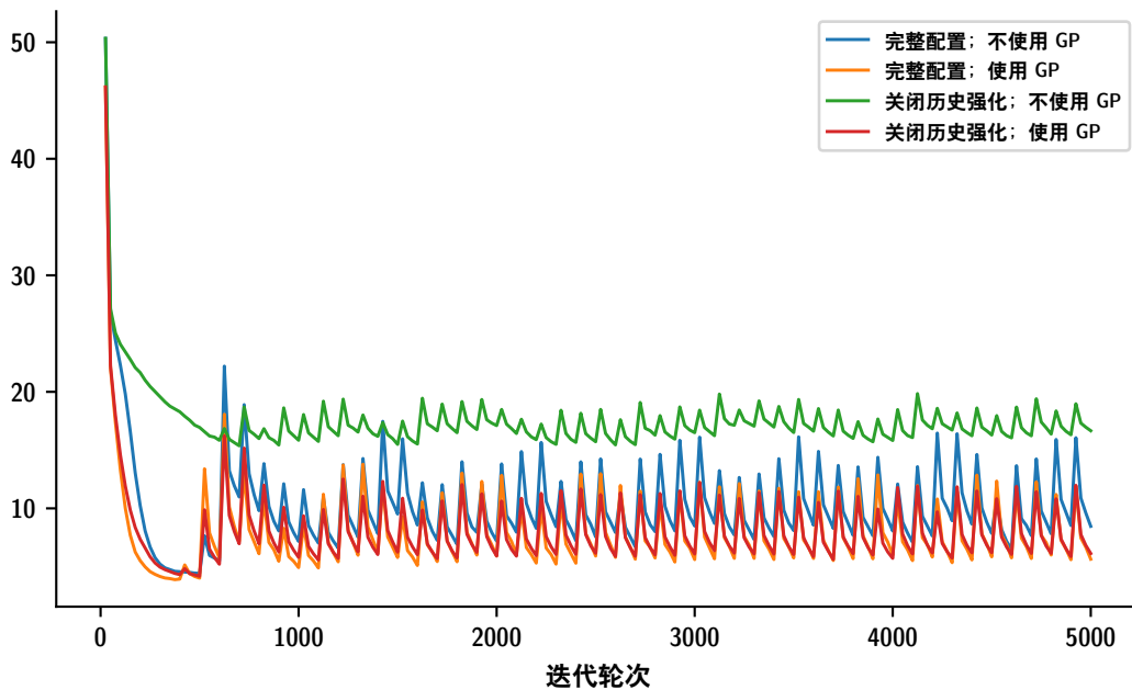
2-opt 后路径之间的边不一致率
