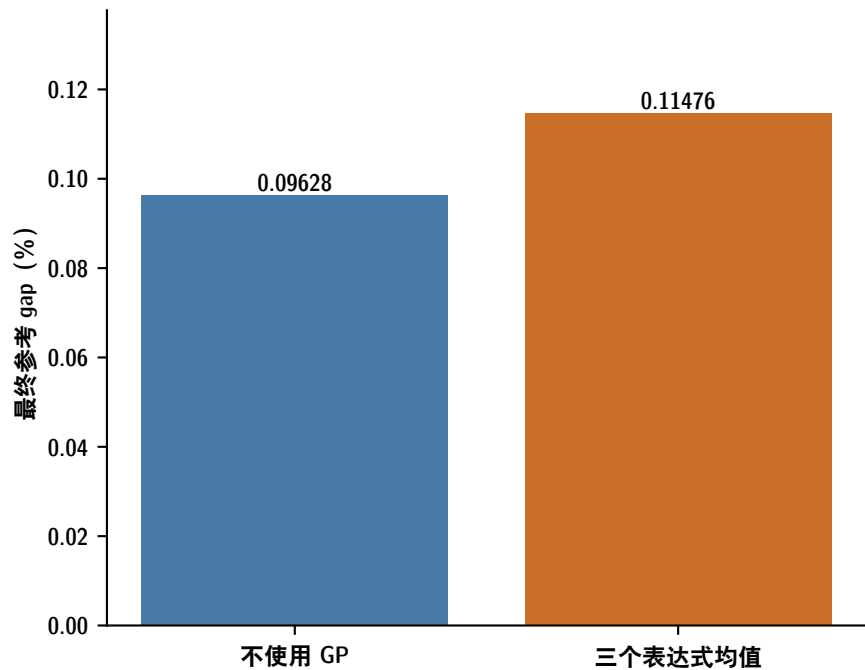
MMAS + 2-opt
