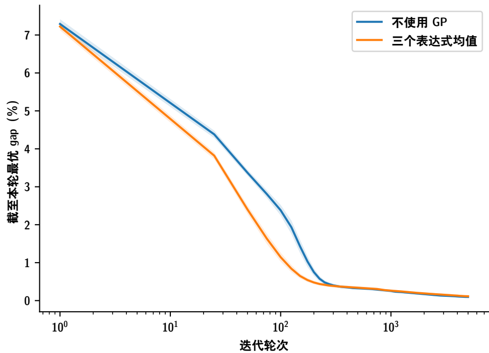
MMAS + 2-opt
