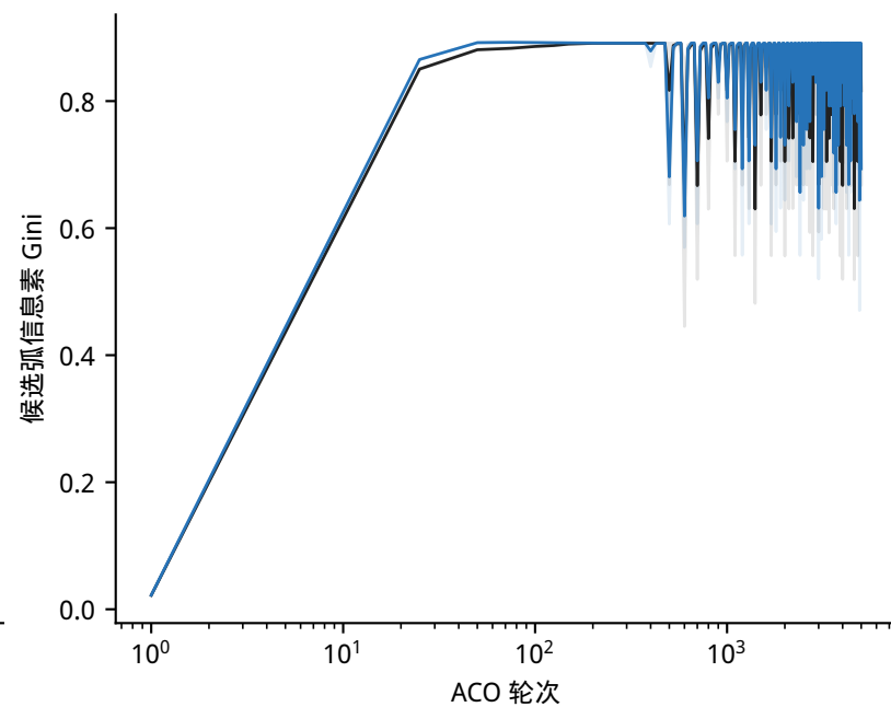
完整 MMAS 中的信息素集中、路径对齐和群体多样性
