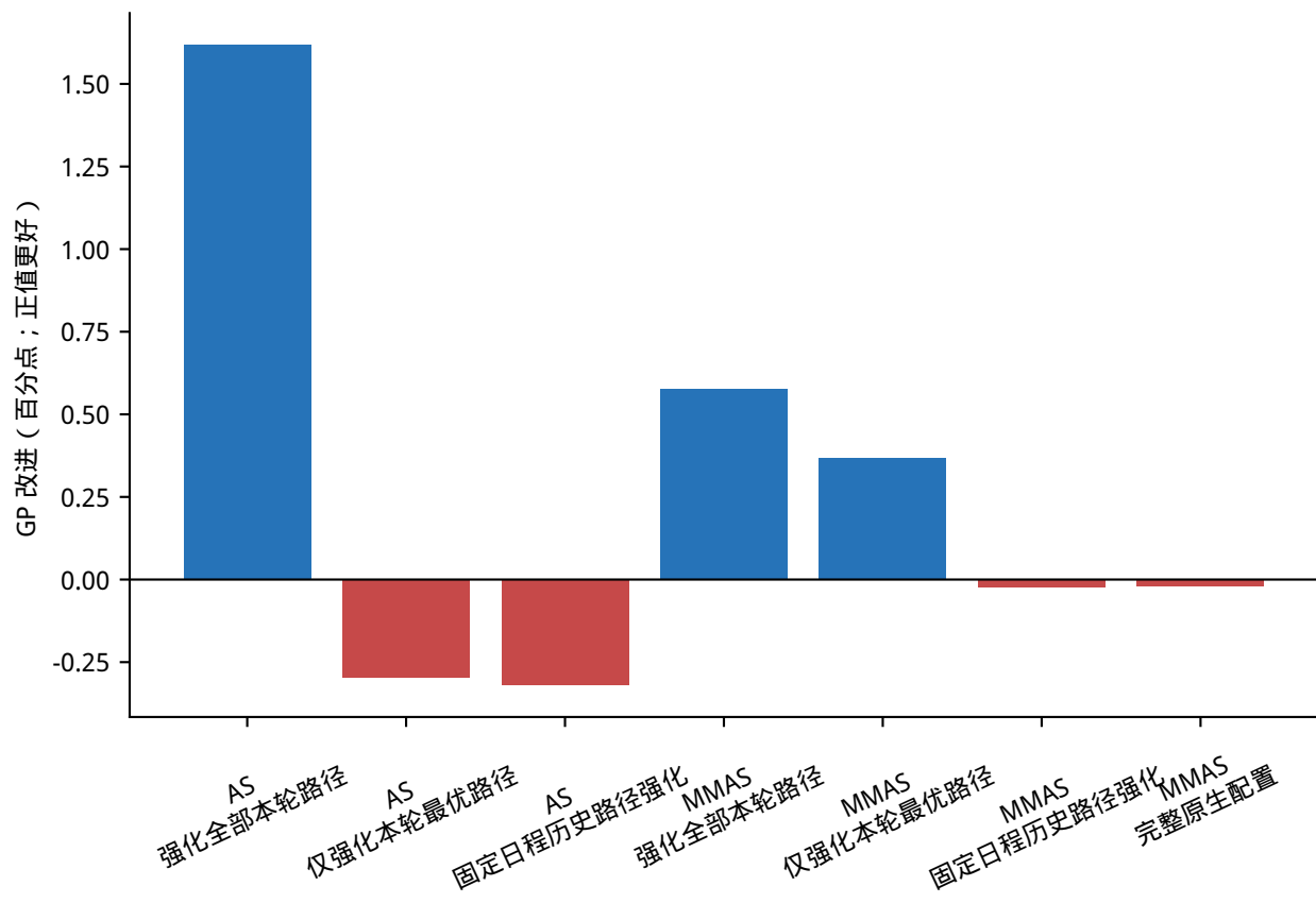
来源越集中于优良路径，GP 的边际空间越小
