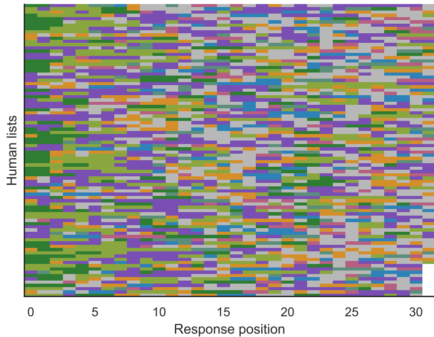
A. Semantic-type trajectories
