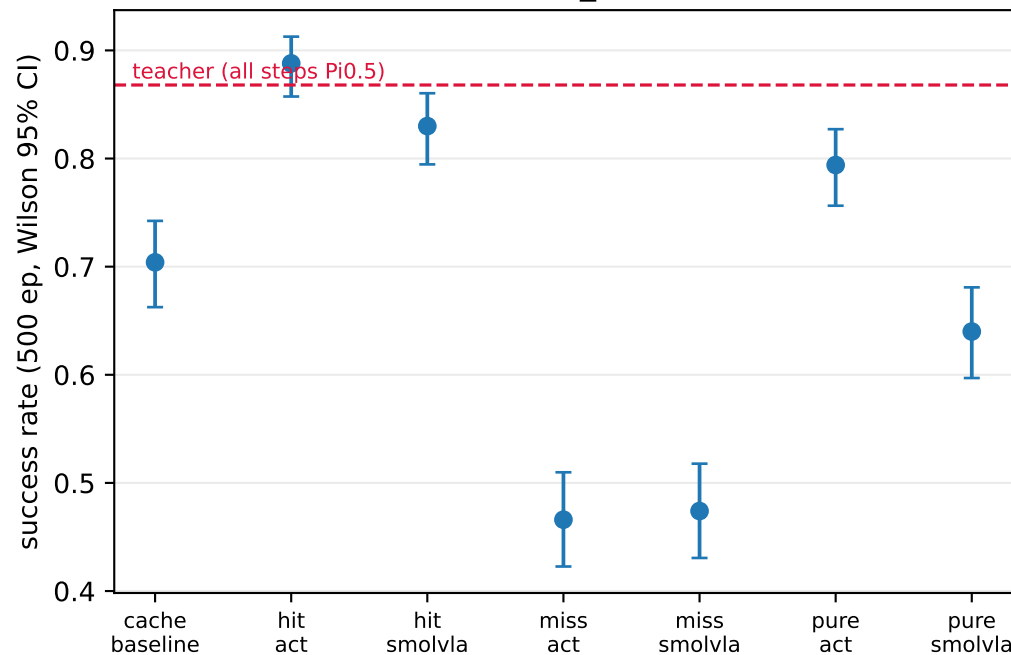
libero_10
