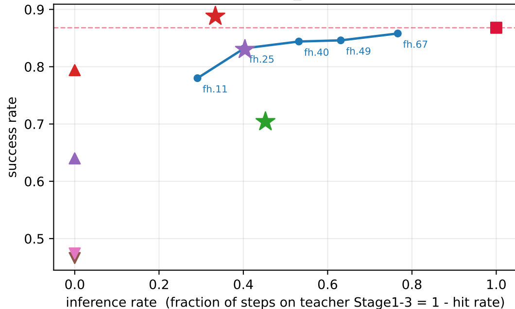
libero_10
