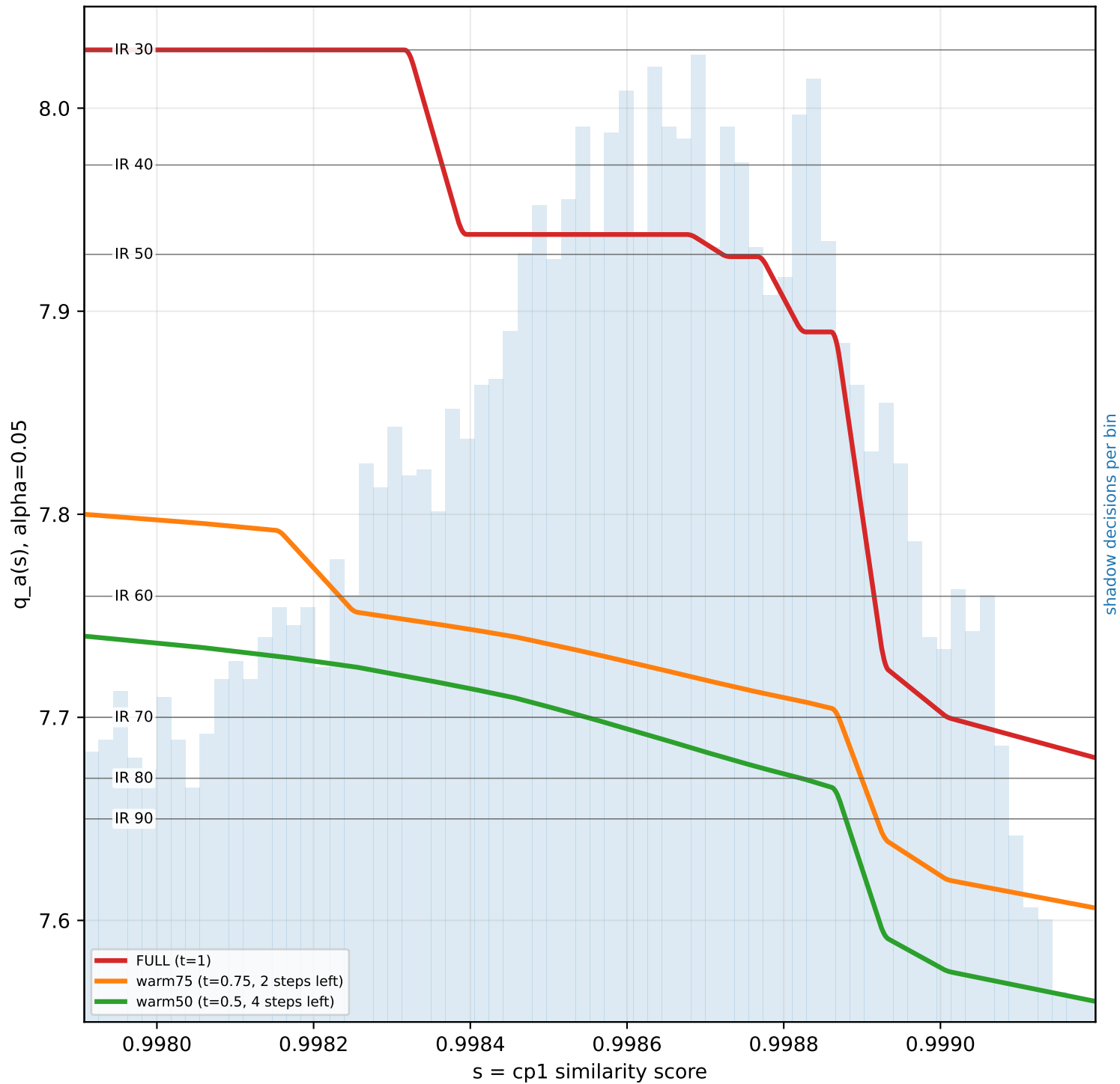
libero_10 K=3
