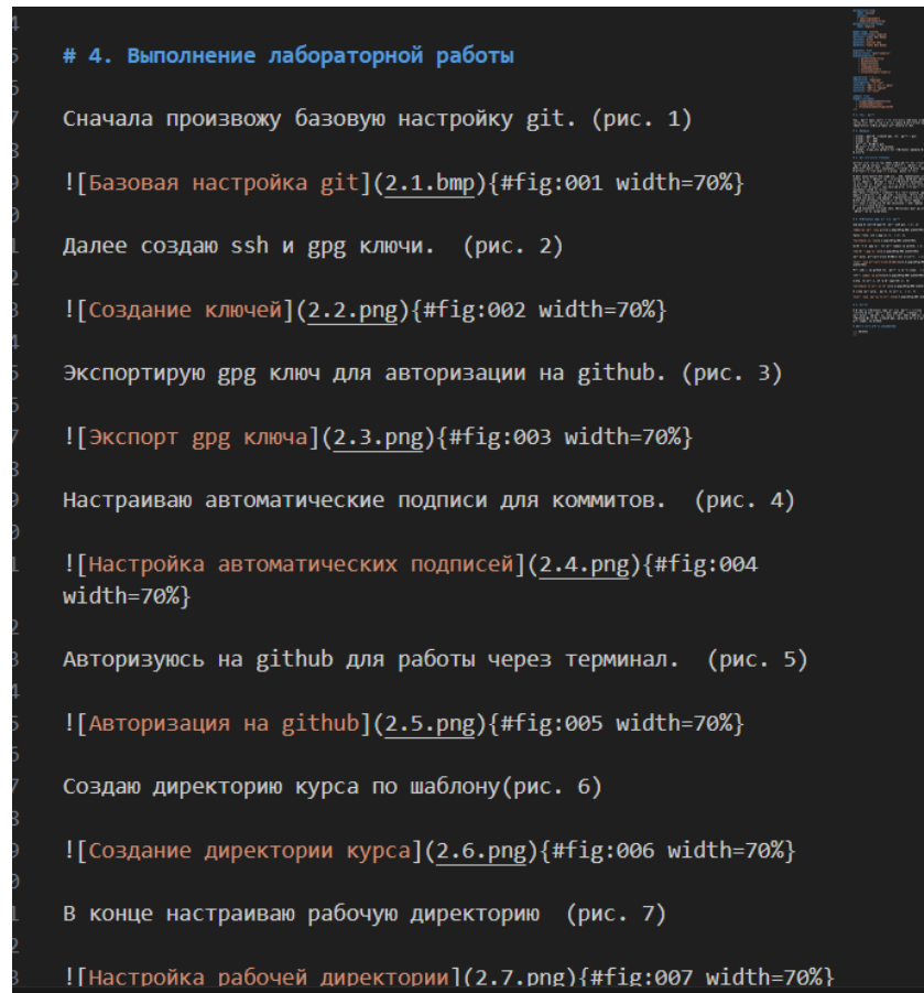
Рис. 3: Процесс выполнения
