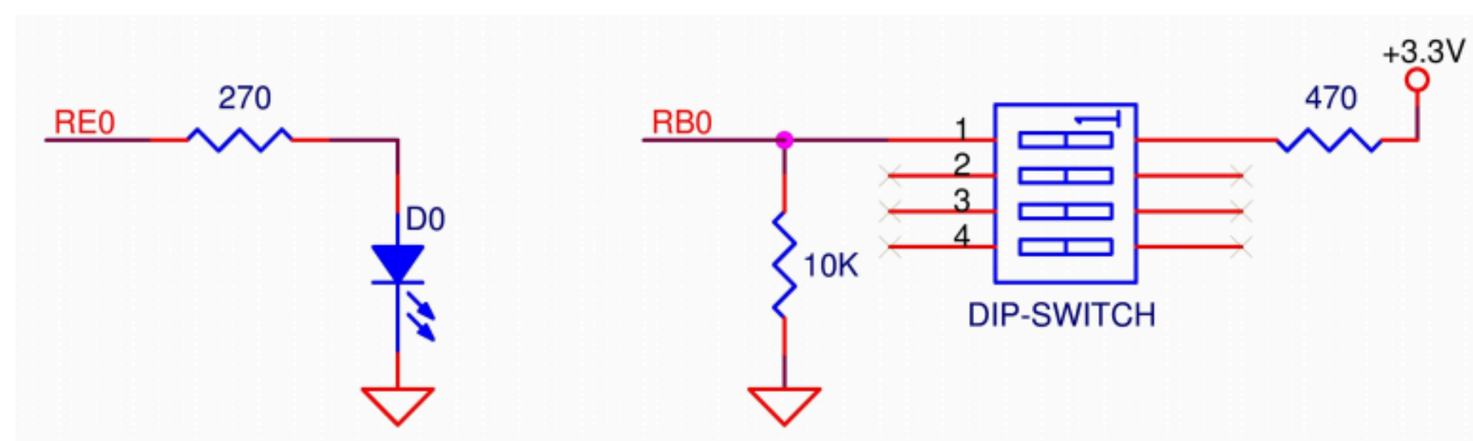
Figura 2. Ligação de um LED e um switch a portos do PIC32.
