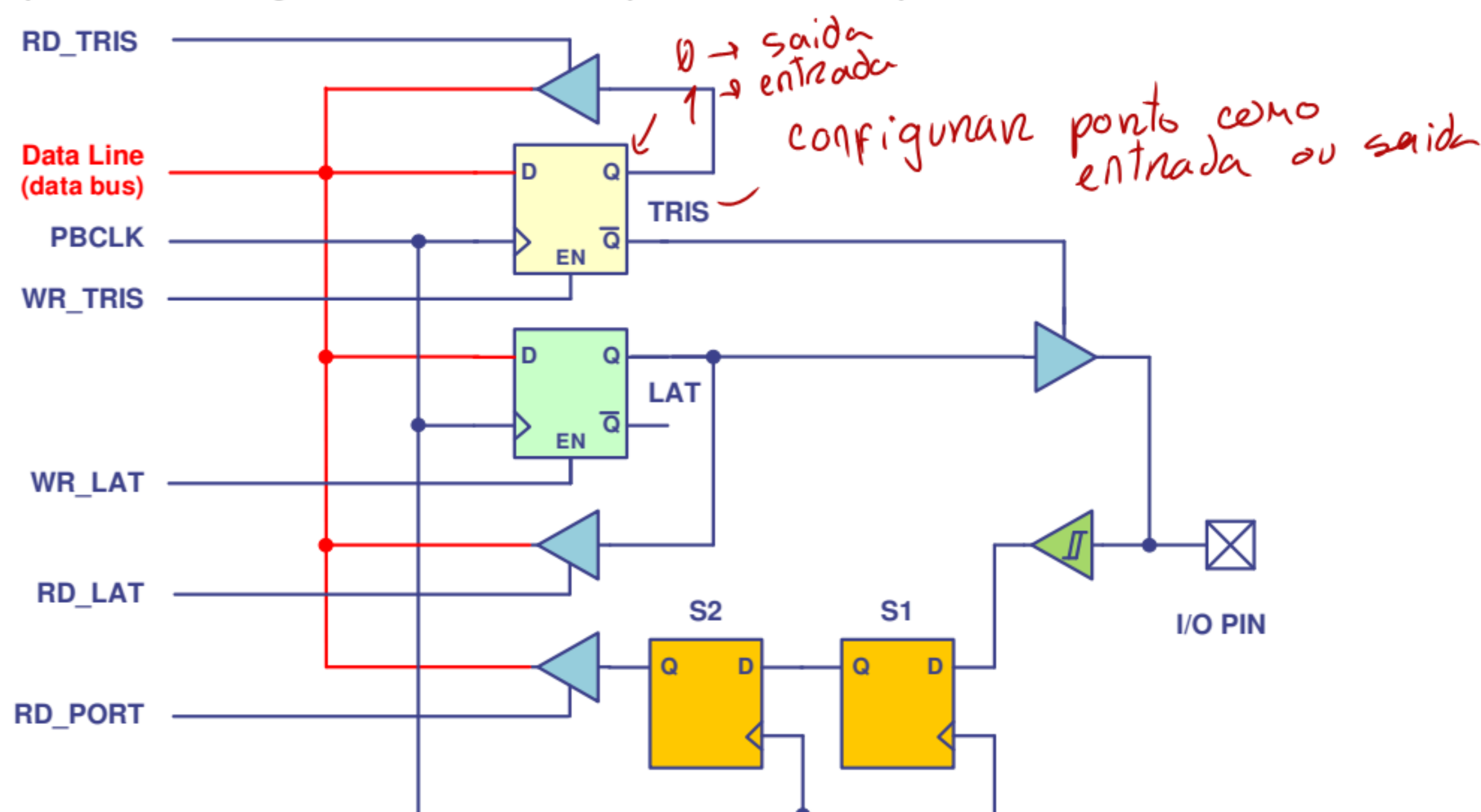
Figura 1. Diagrama de blocos simplificado de um porto de I/O de 1 bit, no PIC32.
