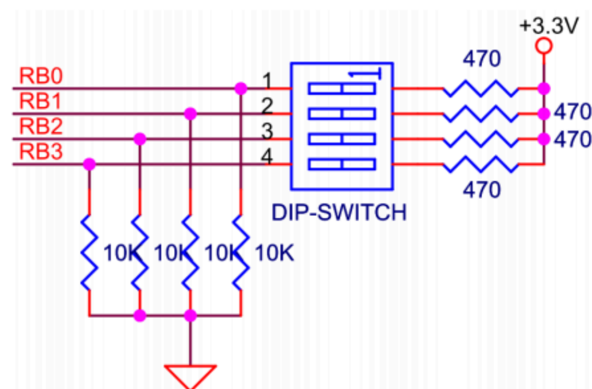
Figura 6. Dip-switch de 4 posições ligado a 4 bits do porto B.
