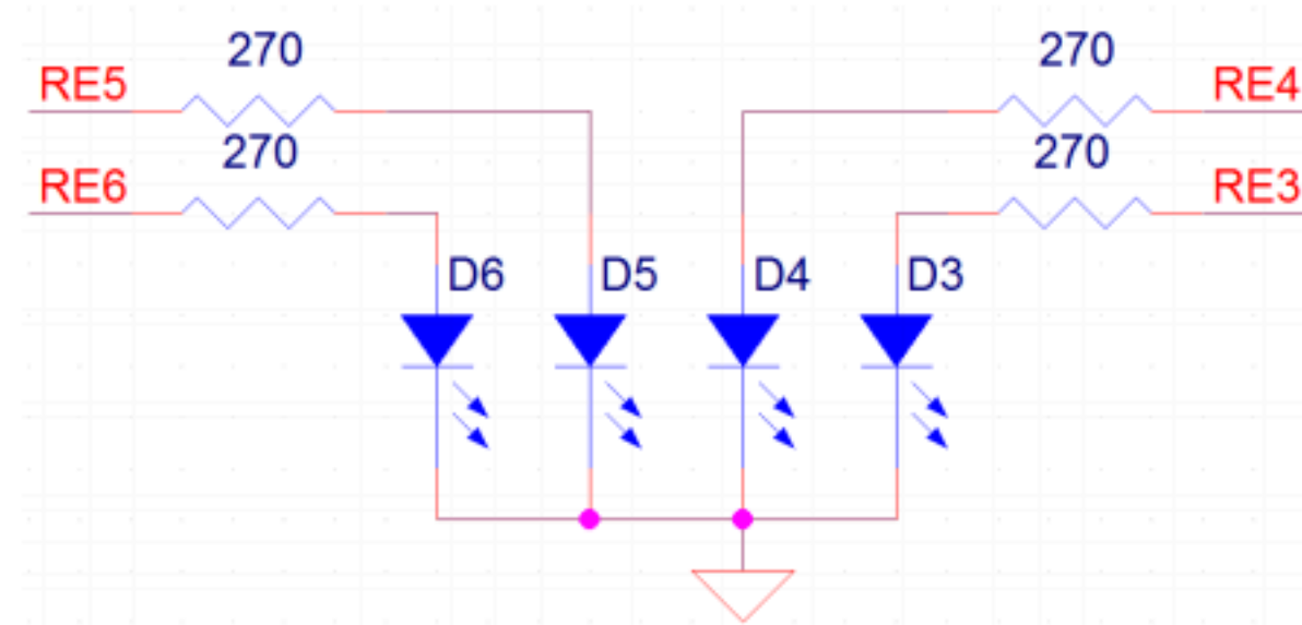
Figura 2. Ligação de 4 LED a portos do PIC32.
