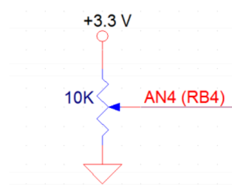
Figura 3. Ligação da resistência variável à placa DETPIC32.
