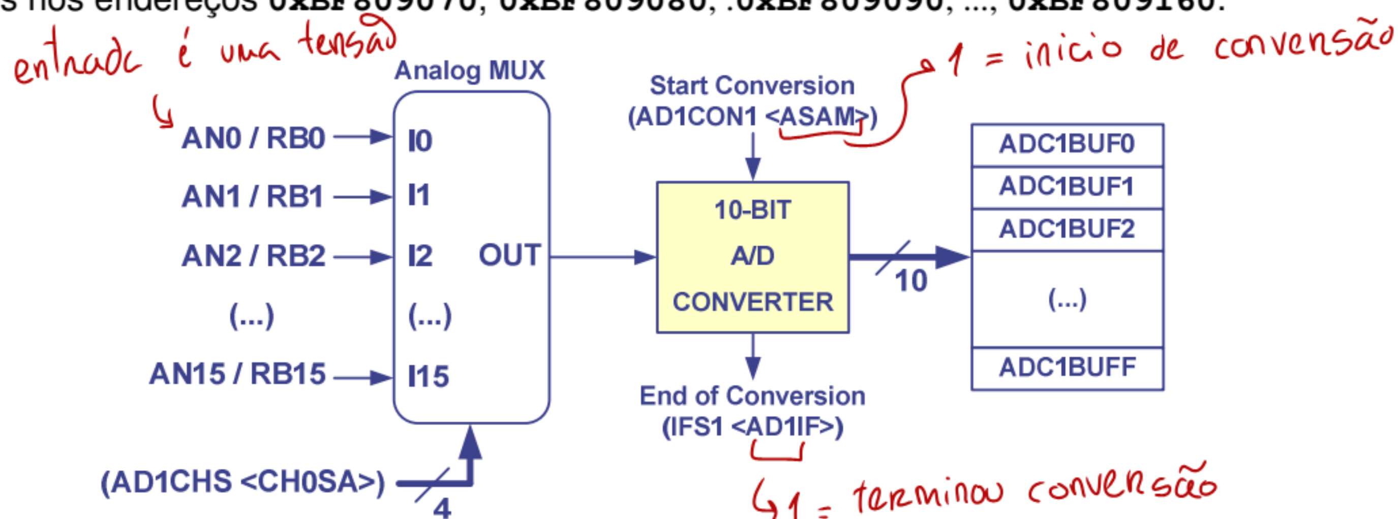
Figura 2. Diagrama de blocos simplificado do módulo A/D do PIC32.
