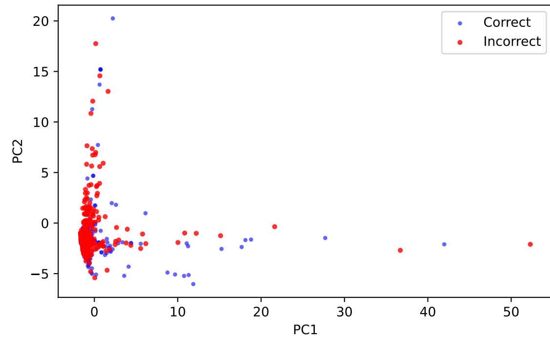
Site 21 — PC1 vs PC2
