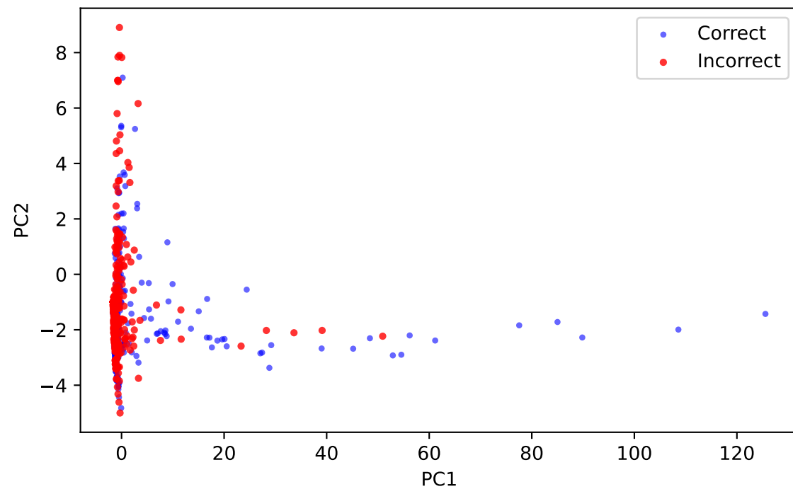
Site 13 — PC1 vs PC2
