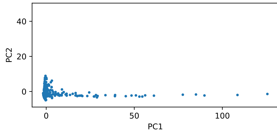
Site 13 — PC1 vs PC2
