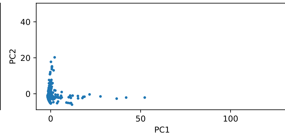
Site 6 — PC1 vs PC2
