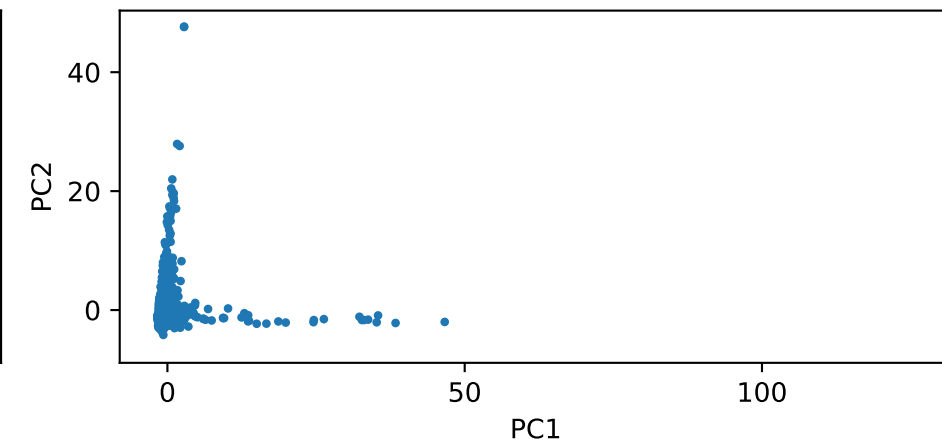
Site 21 — PC1 vs PC2
