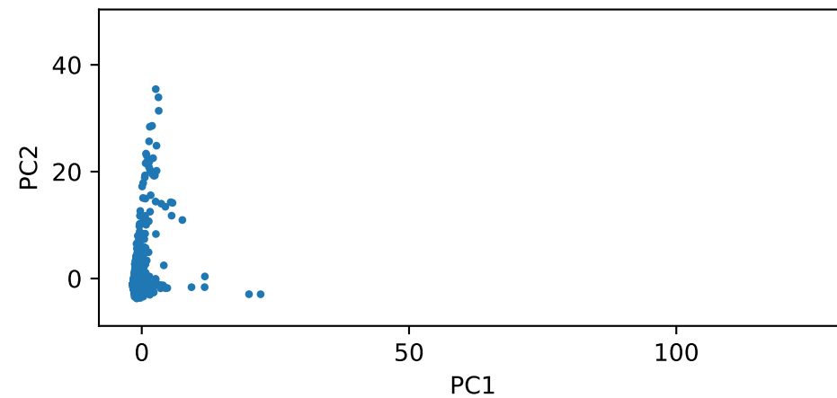
Site 4 — PC1 vs PC2
