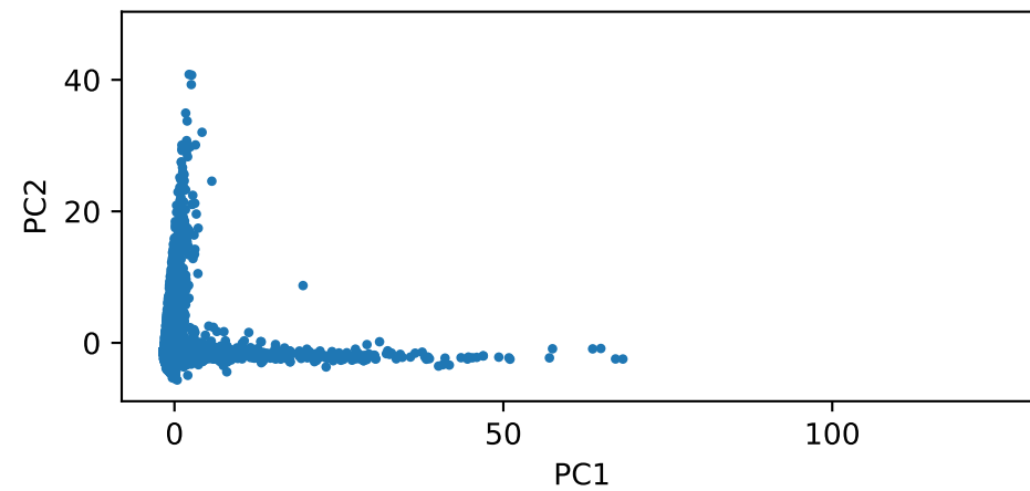
Site 18 — PC1 vs PC2
