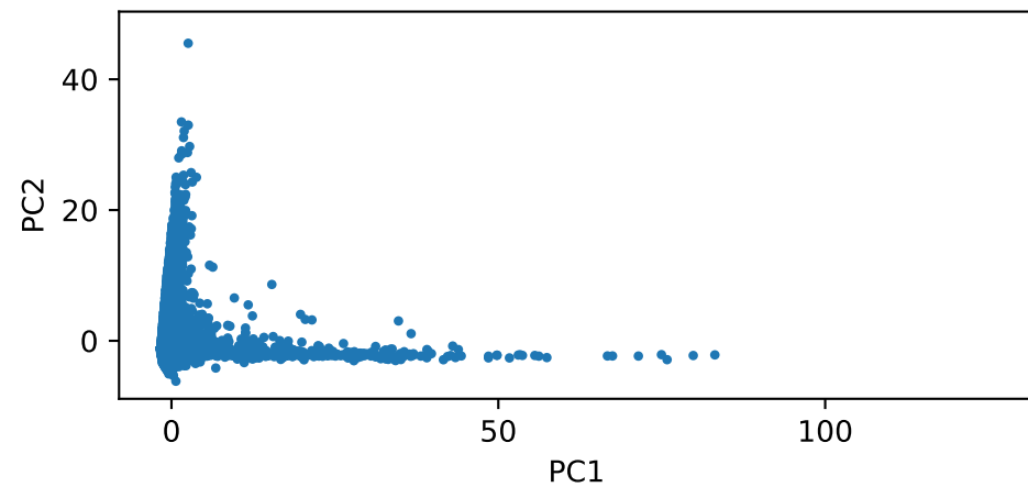
Site 1 — PC1 vs PC2
