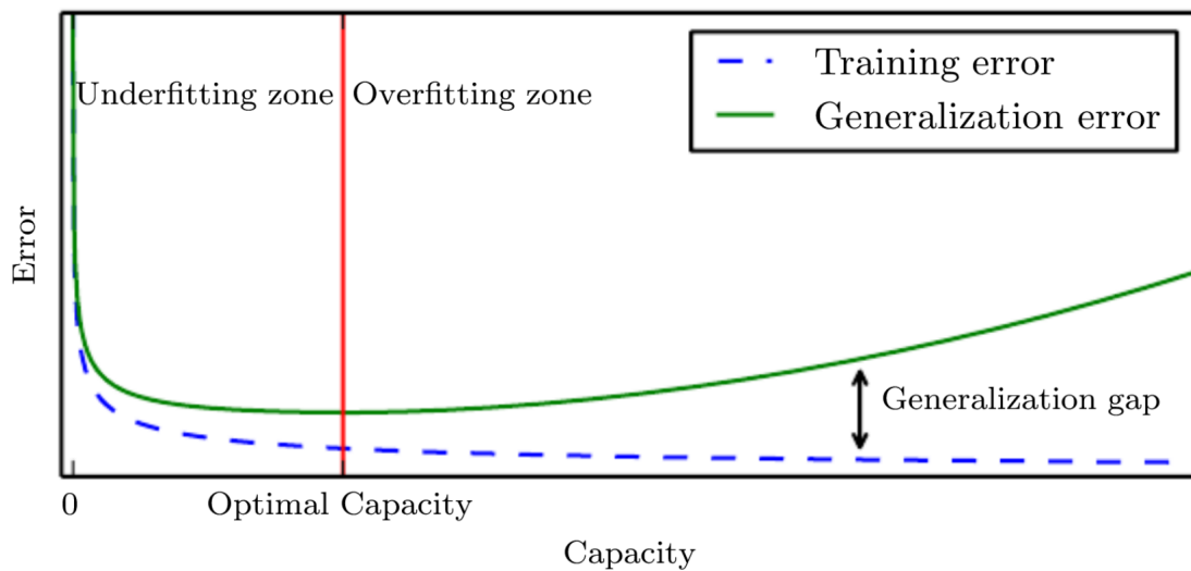
图 10.7 模型容量与训练误差、泛化误差之间的示意关系。横轴是容量, 不是训练轮次。
