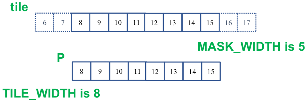
图 9.3 8 个连续输出对应 12 个不同输入。左右各两个光环元素保证最外侧输出也能获得完整的五点窗口。
