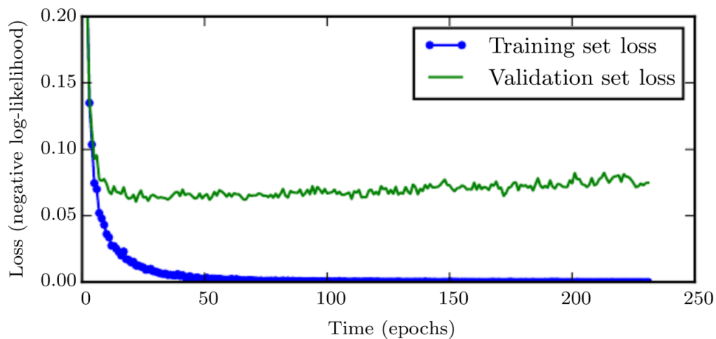
图 10.6 训练损失与验证损失随训练轮次的变化。纵轴为负对数似然损失；该曲线用于说明泛化现象，与前面数字距离损失的数值例题分开讨论。
