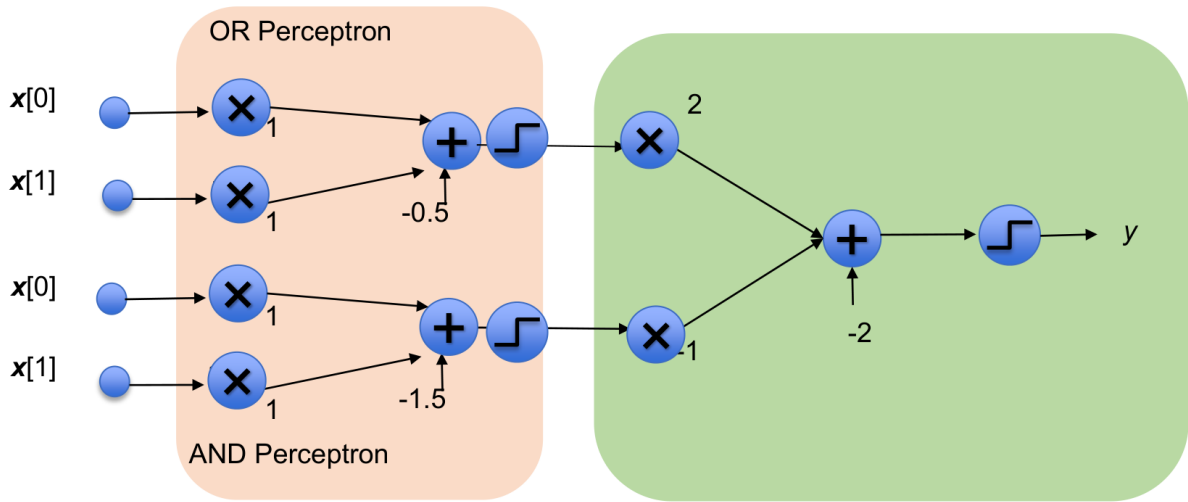
图 10.3 OR 与 AND 感知机构成隐藏层，再由带权组合和符号函数给出 XOR 输出。乘号旁的数值是连接权重，加法器旁的常数是偏置。
