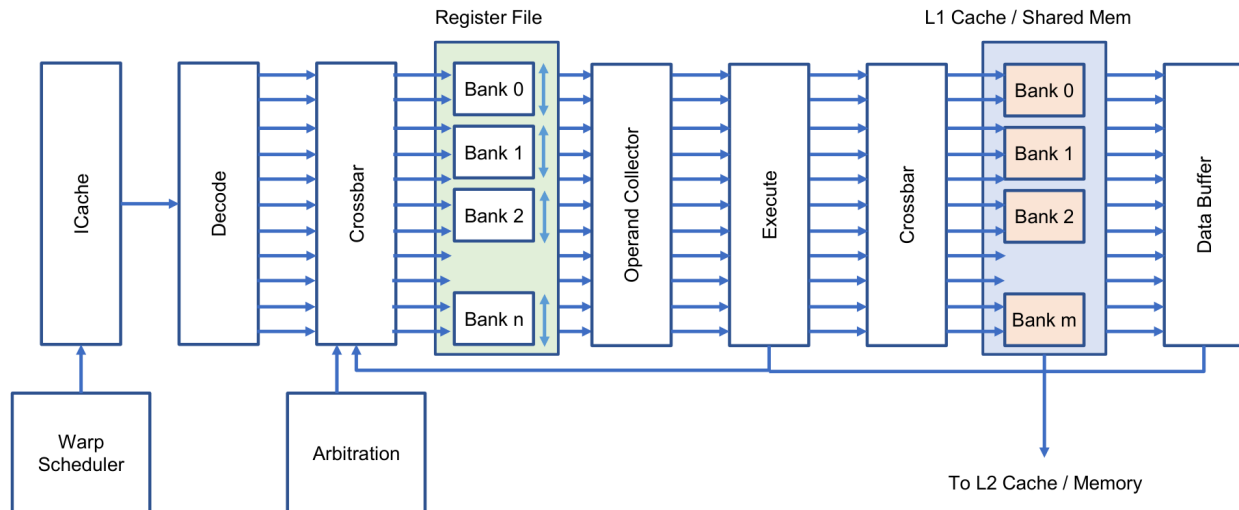
图 9.6 概念性的 SM 执行流水线。寄存器文件与 L1 / 共享内存均采用多存储体组织，交叉开关连接执行通路、操作数收集与存储通路。
