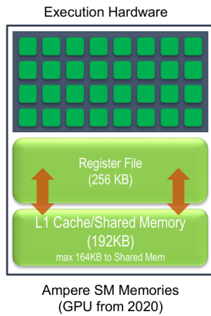
图 9.5 A100 示例中的片上存储容量及粗略访问层次。线程容量与共享内存容量共同限制可驻留线程块的数量。
