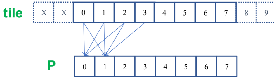
图 9.4 左边界输入分块中的两个虚拟位置。它们占用共享内存位置，但不需要从输入数组加载。
