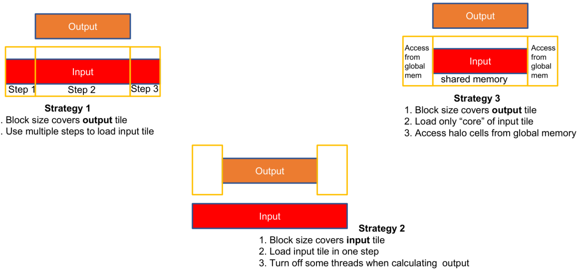
图 9.1 三种策略的加载范围与线程分工。策略 1 分多步装入完整输入，策略 2 为完整输入分配线程，策略 3 仅将核心区置于共享内存。
