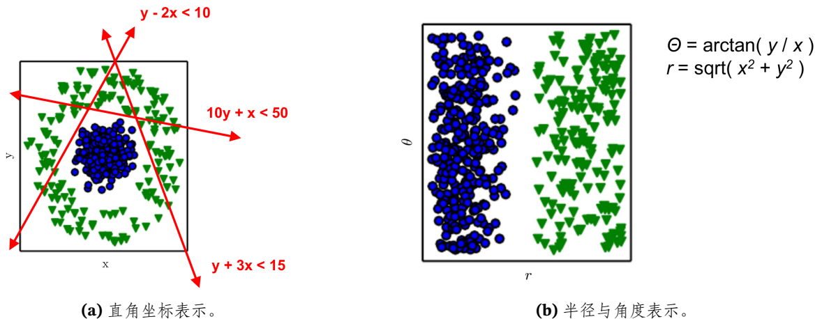
图 10.1 相同分类任务在不同特征坐标下具有不同的分离难度。
