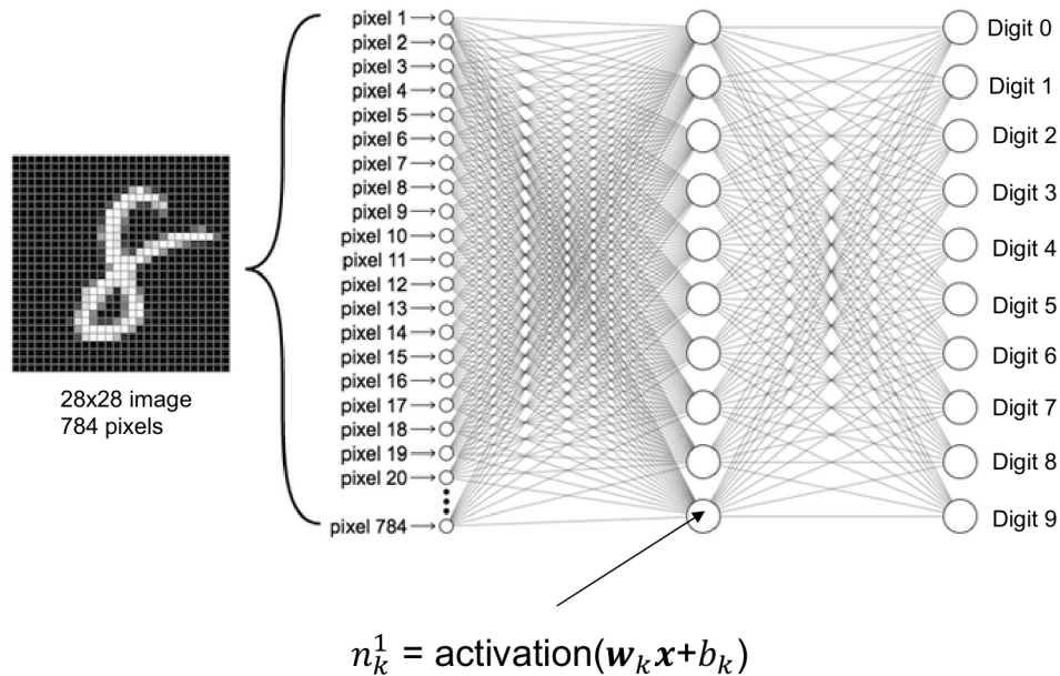
图 10.4 784 → 10 → 10 的手写数字识别网络。每个隐藏单元对 784 个像素加权求和，并经过激活函数；输出端有 10 个类别分量。
