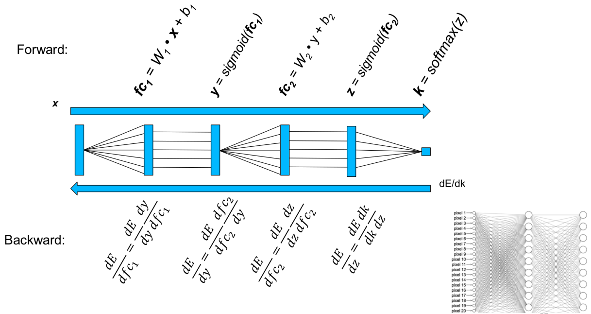
图 10.5 前向从输入逐层计算至概率输出，反向从损失对概率的导数逐层向前传播。图中的第二层也包含 sigmoid。
