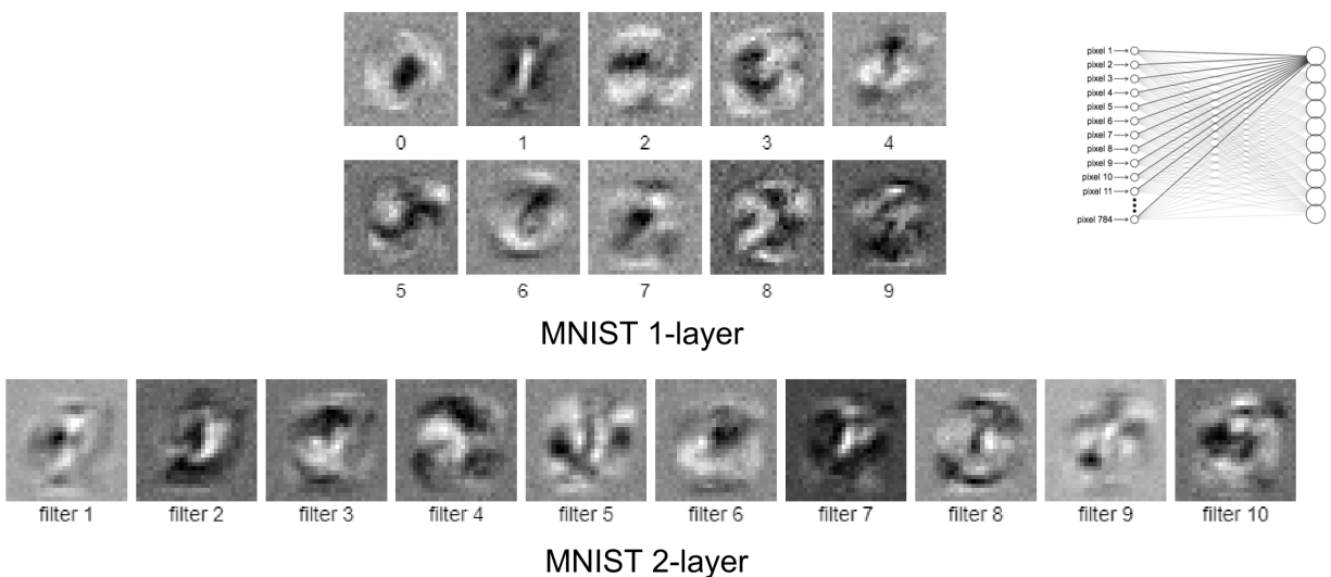
图 10.8 单层 MNIST 网络的类别权重图与两层网络的特征权重图。上方以数字 0-9 标注，下方以特征编号标注。
