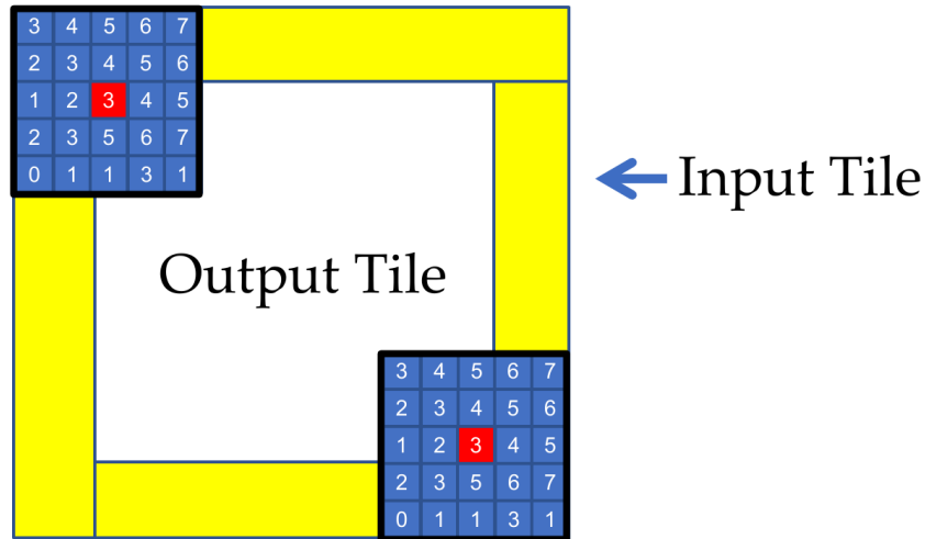
图 9.2 计算输出分块两个相对角点时，其输入窗口分别延伸到左上与右下的光环区域。白色输出区域外的黄色边框也是输入分块的一部分。
