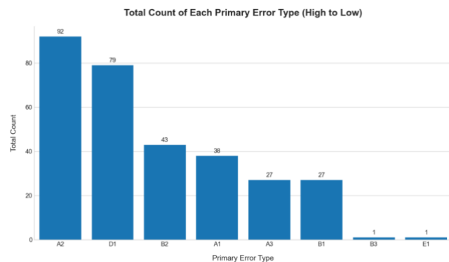
(d) GPT error distribution
